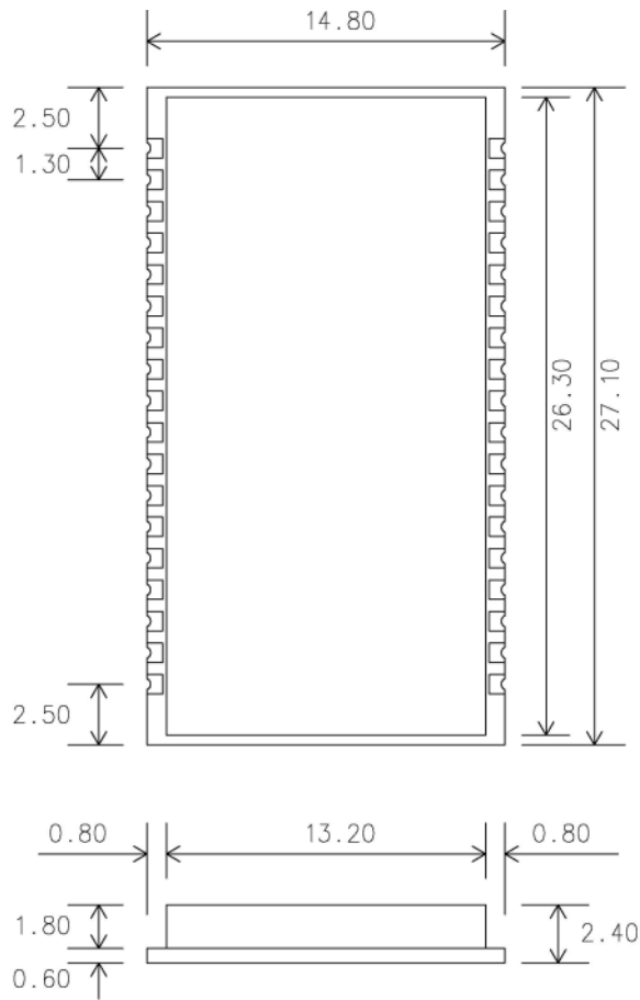
그림 1-3 모듈 치수
