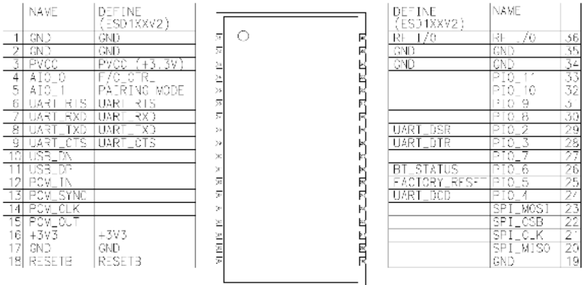
그림 1-2 핀 배치도
