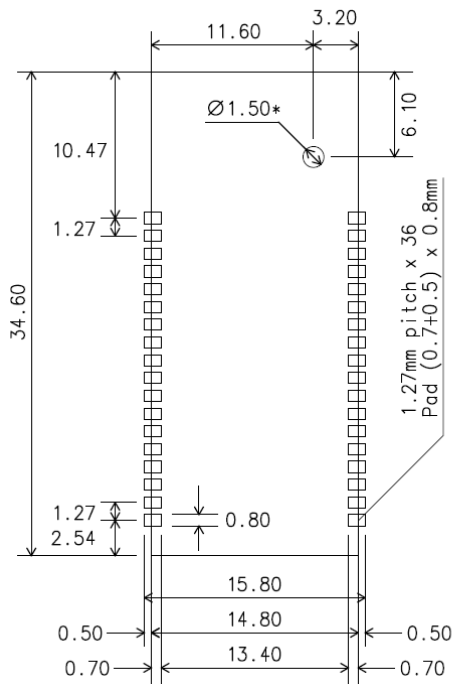
[SMD 타입]
