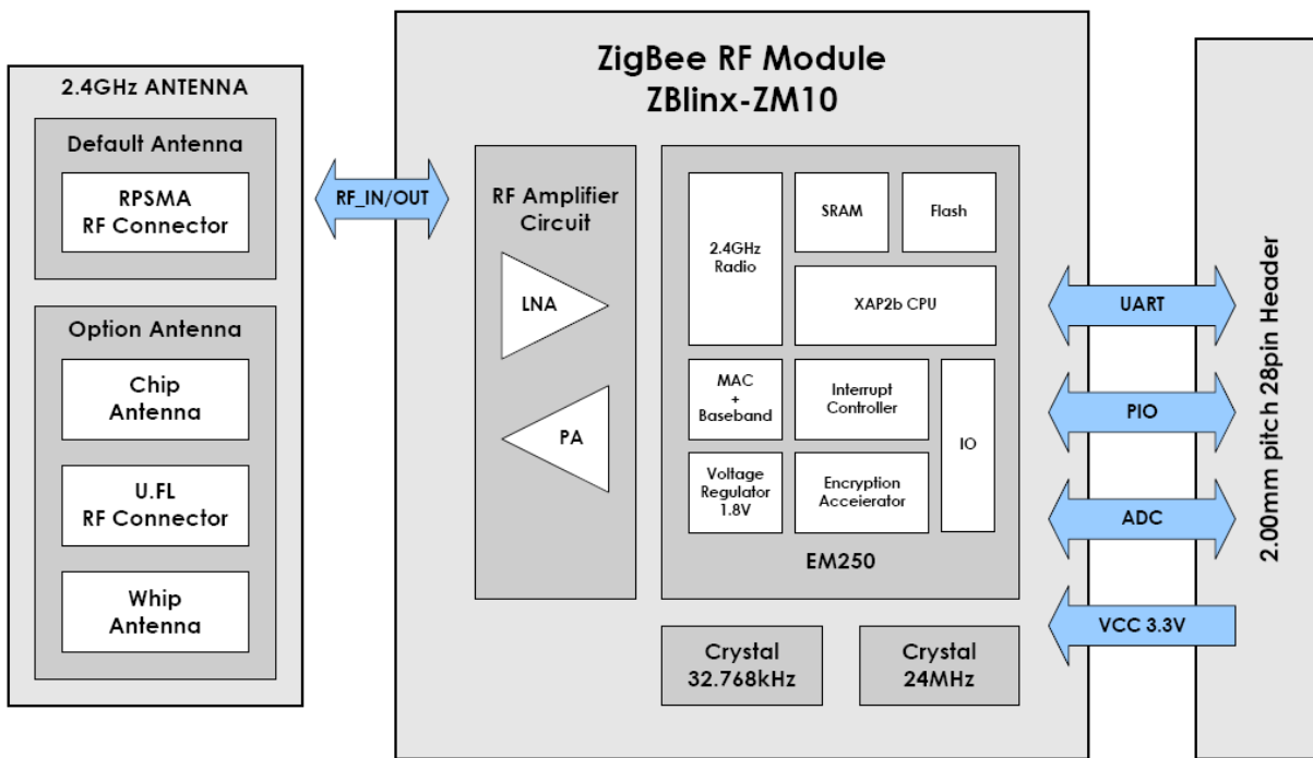
그림 1-1 블록 다이어그램
