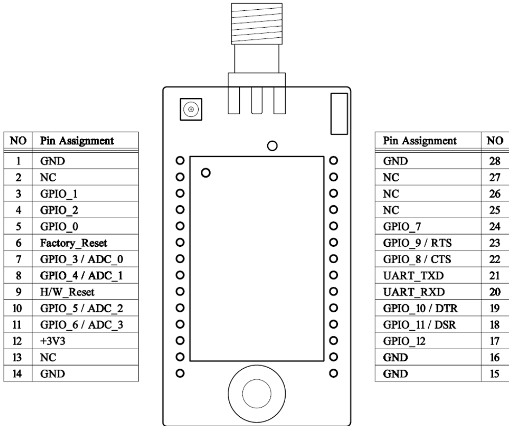
그림 1-2 핀 배치도
