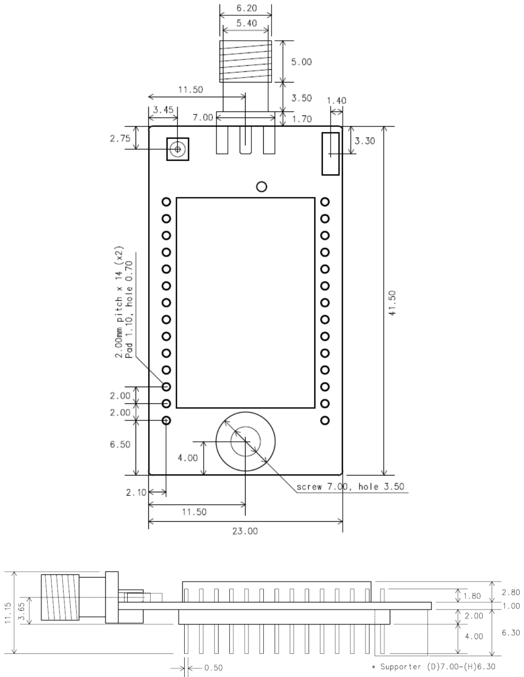
그림 1-3 치수도
