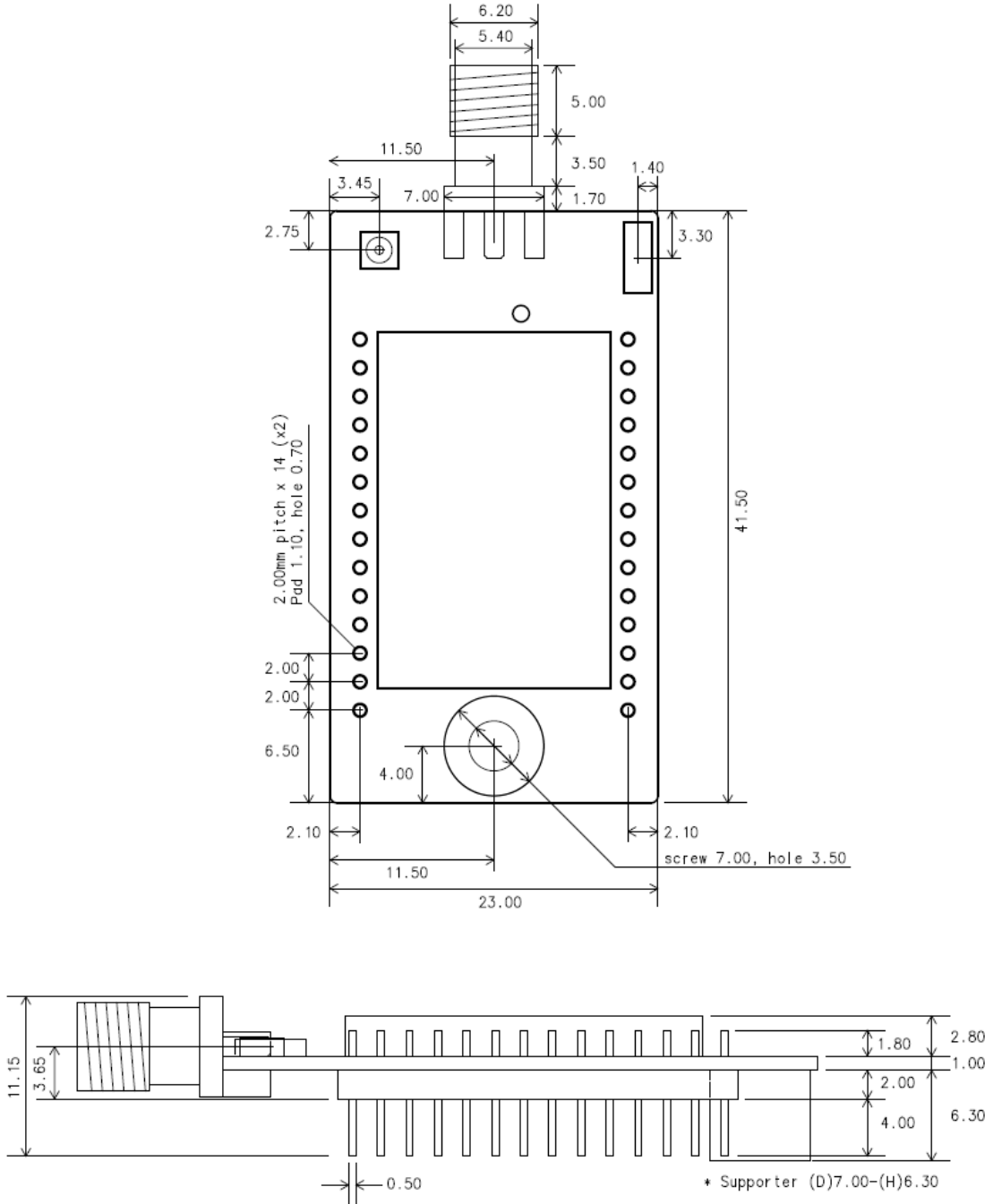
그림 1-3 치수도
