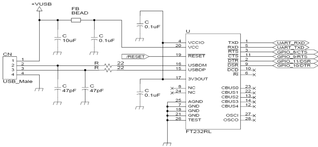
그림 5-4 USB-UART 변환
