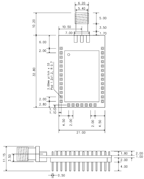
그림 1-4 ProBee-ZE20SDS 치수도
