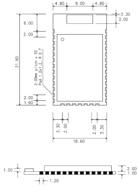
그림 1-7 ProBee-ZE20SSC 치수도
