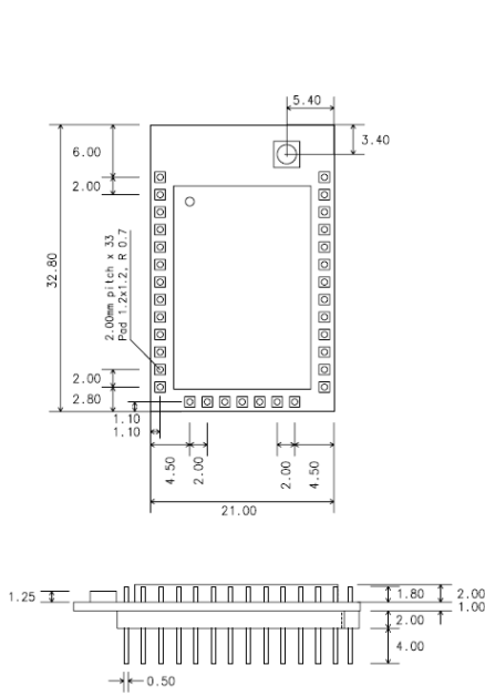
그림 1-3 ProBee-ZE20SDU 치수도
