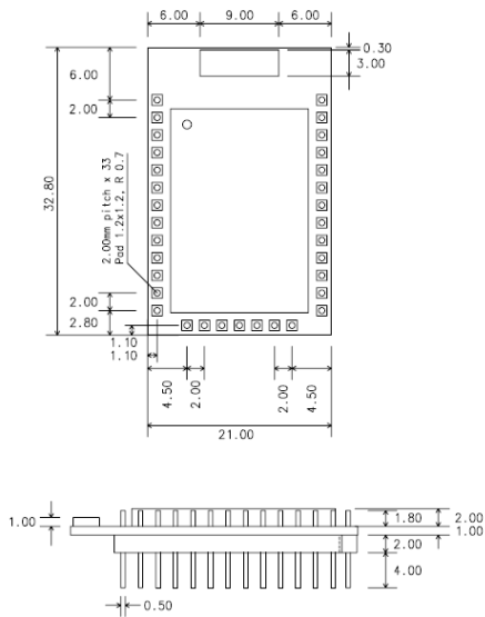
그림 1-5 ProBee-ZE20SDC 치수도
