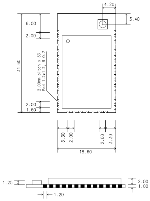
그림 1-6 ProBee-ZE20SSU 치수도
