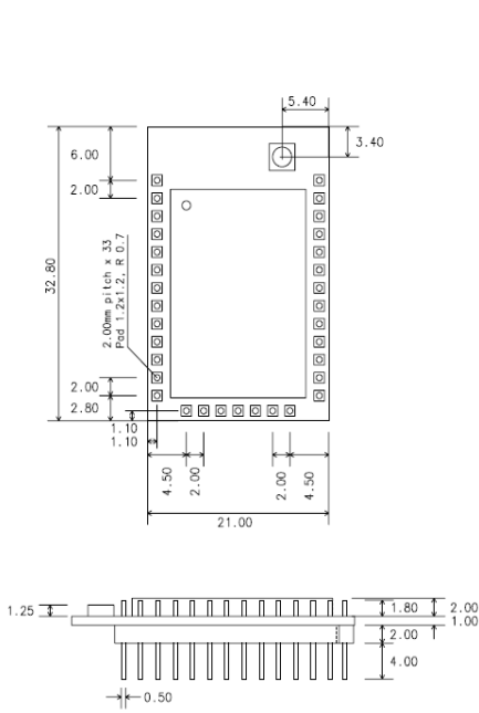
그림 1-3 ProBee-ZE20SDU 치수도
