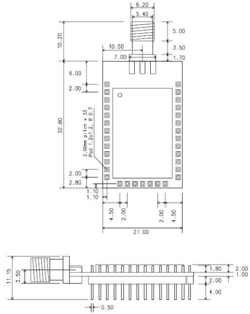
그림 1-4 ProBee-ZE20SDS 치수도
