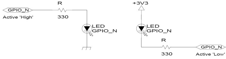
그림 5-6 GPIO LED 출력
