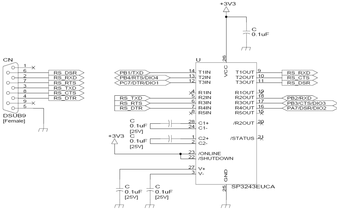
그림 5-3 RS232 시리얼
