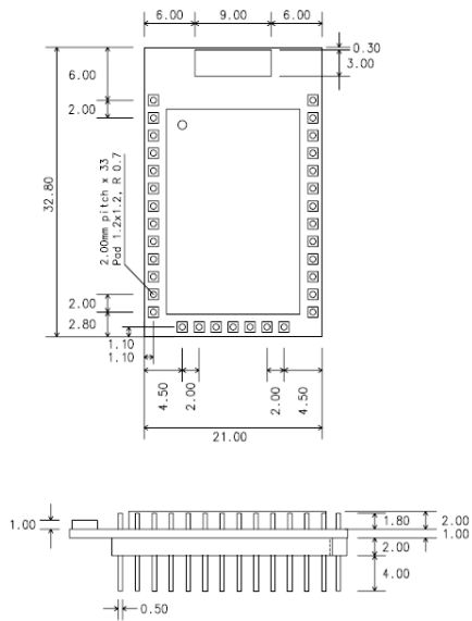
그림 1-5 ProBee-ZE20SDC 치수도
