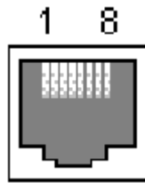
Figure A-1 RJ45 Ethernet 커넥터의 핀 배치
