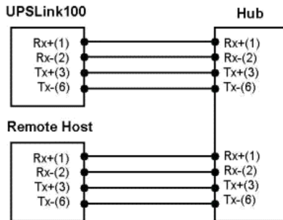
Figure A-4 다이렉트 Ethernet 케이블을 이용한 Host간 간접 연결
