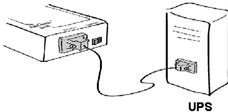
Figure 2-4 UPSLink에 UPS를 연결하기
