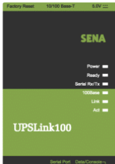
Figure 2-1 UPSLink 100의 패널 배치
