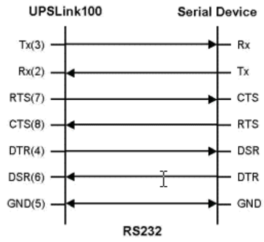
Figure A-5 RS232 결선도
