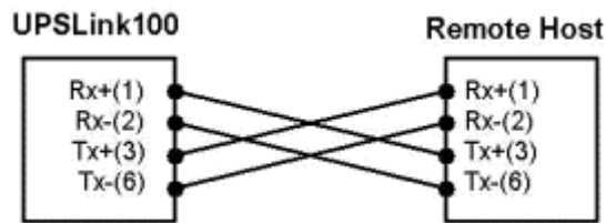
Figure A-3 크로스 Ethernet 케이블을 사용한 Host간 직접 연결
