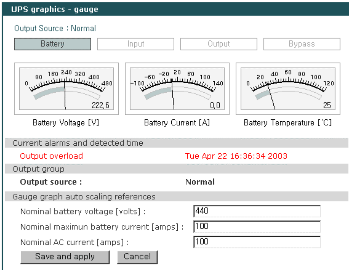
Figure 3-4 UPS 게이지 그래픽
