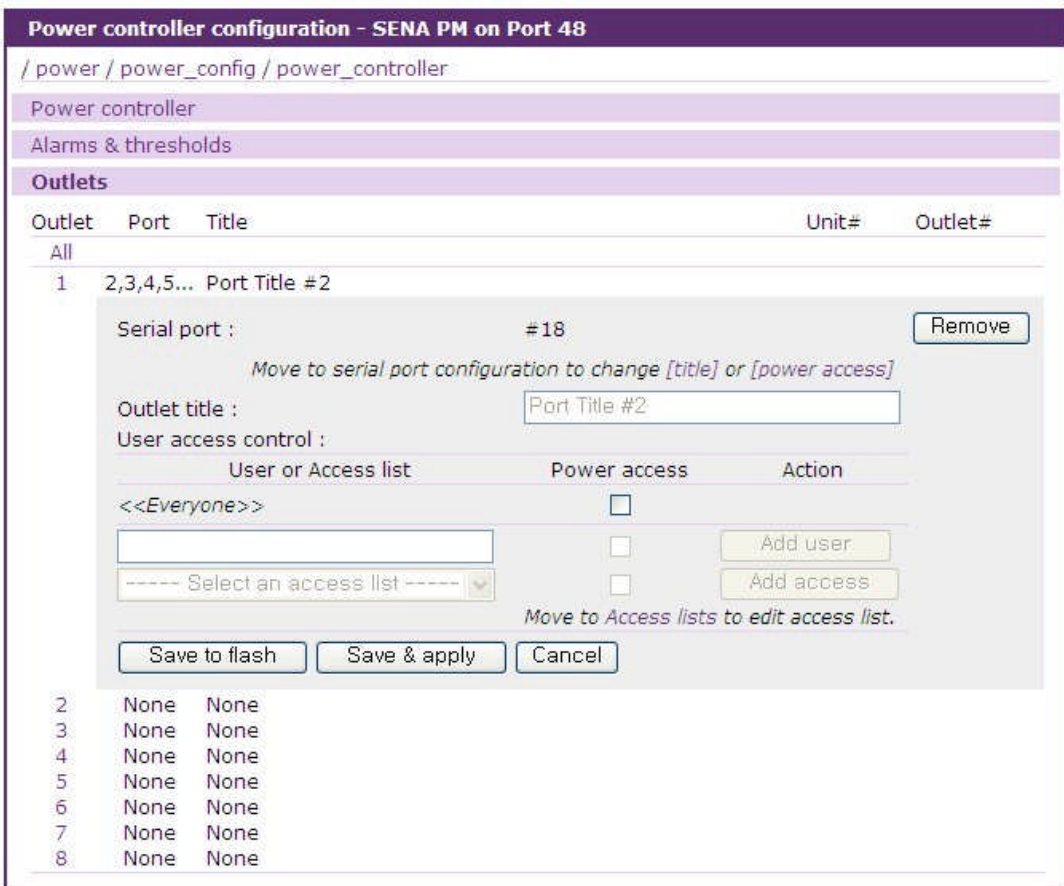
그림 6-9 파워 컨트롤러 유닛 설정 - 아웃렛 설정 - 링크된 시리얼 포트 설정
