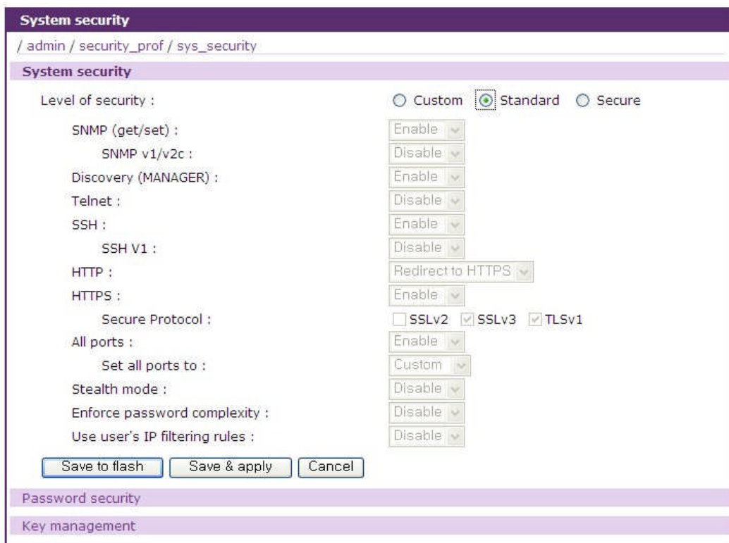
그림 9-11. Security profile – System security
