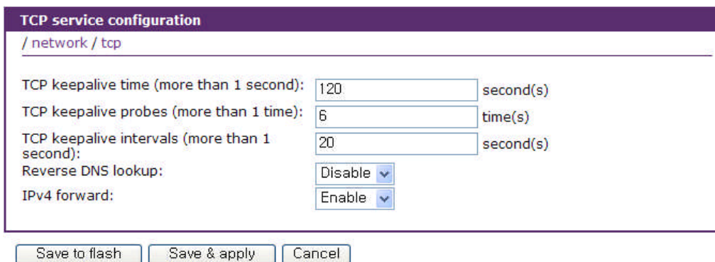
그림 3-13 TCP service 설정
