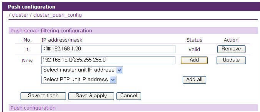
그림 5-23 Push server filtering configuration with setting IP address manually
