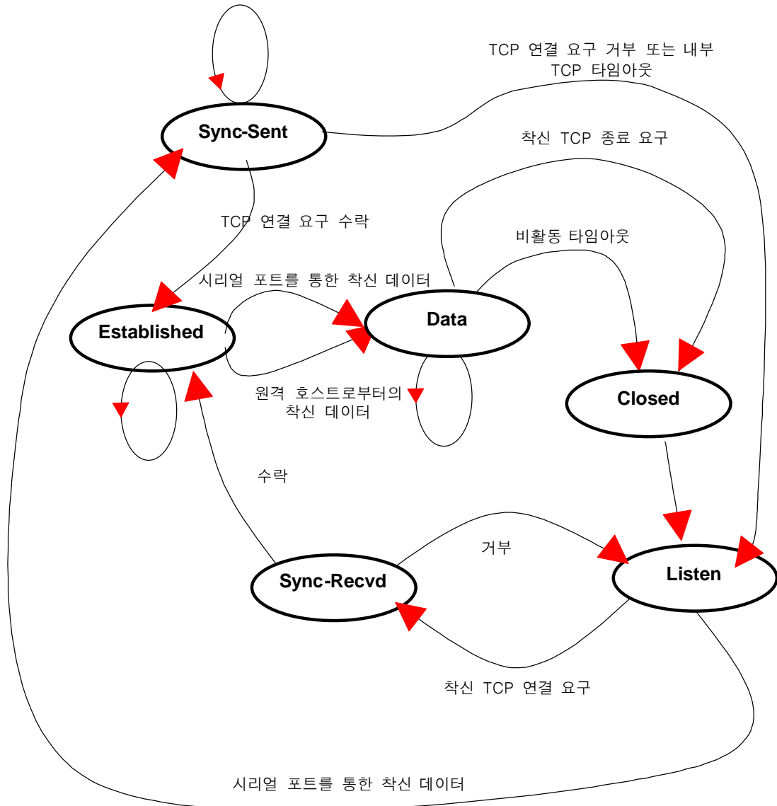
그림 5-5. TCP 서버/클라이언트 모드의 상태 전이도
