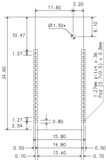
[SMD 형]
