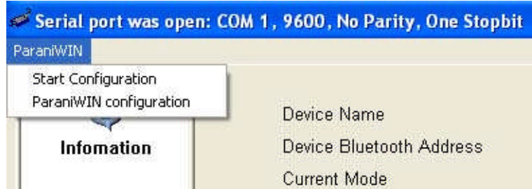
그림 3-4 ParaniWIN 메뉴
