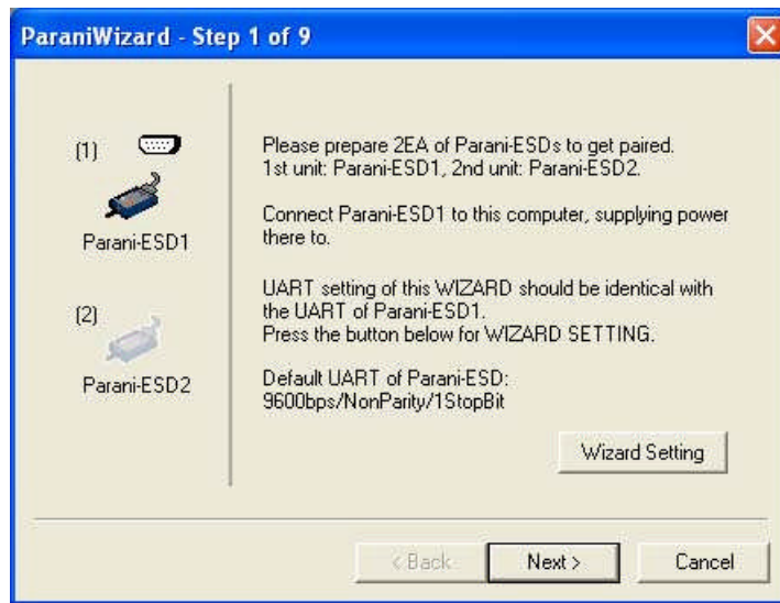
그림 3-10 ParaniWizard Step 1
