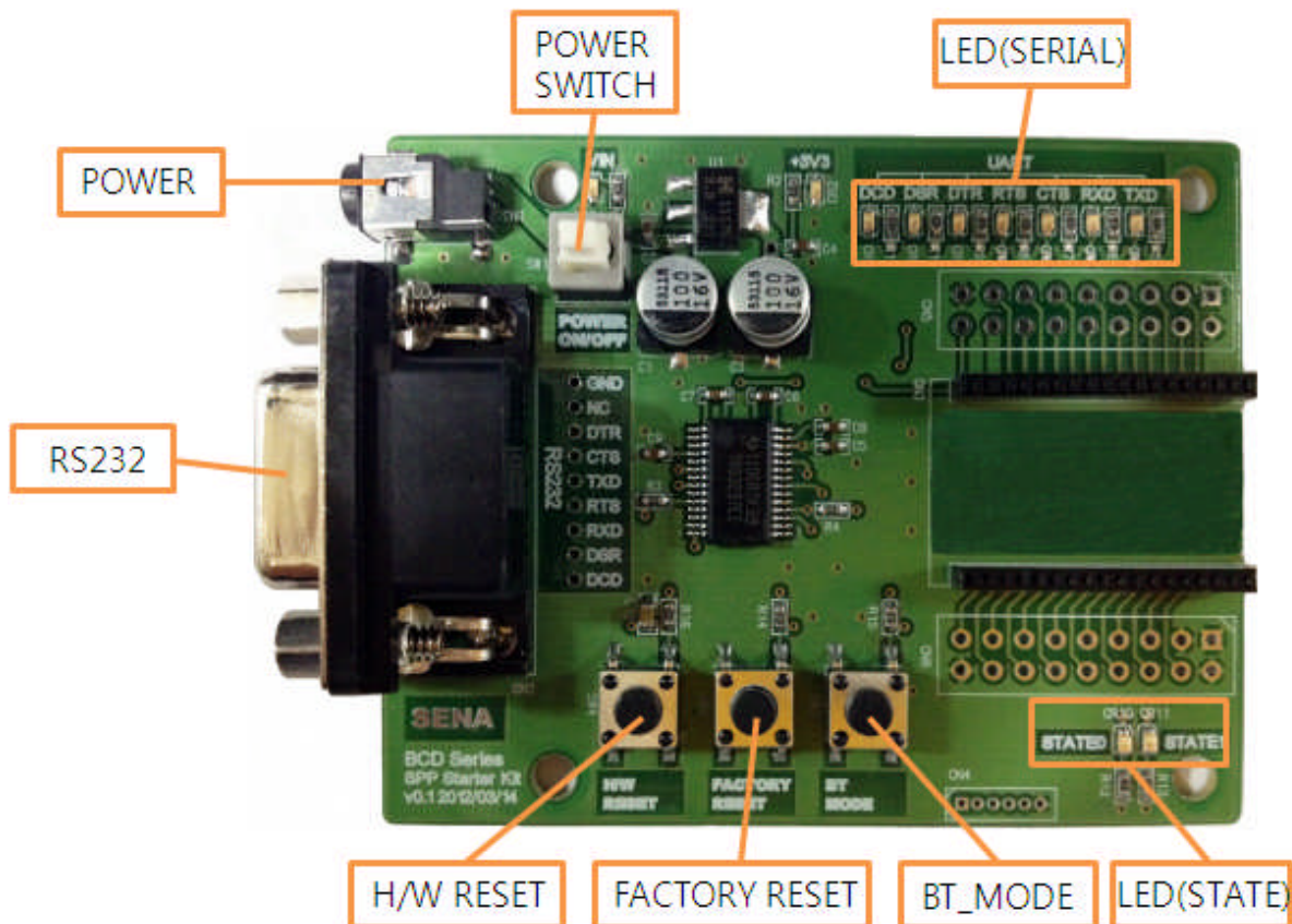
그림 Error! Style not defined.-1 BCD 개발 보드 패널 배치
