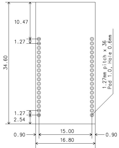
[DIP 형]
