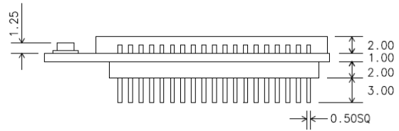
[BCD110DU]
