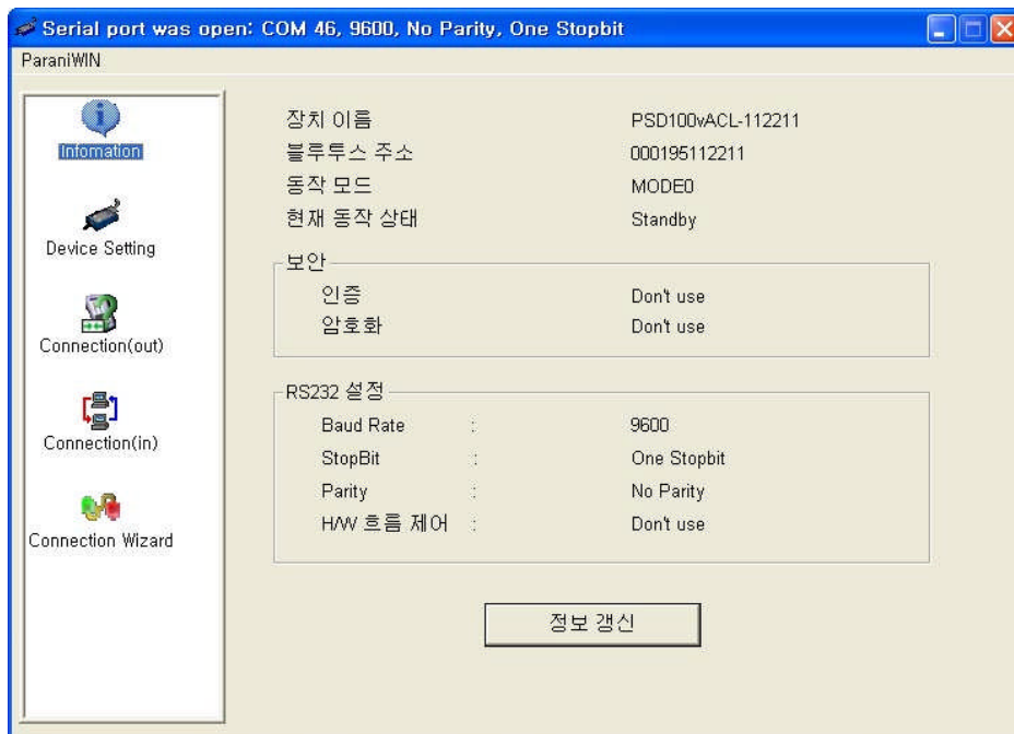
그림 3-3 Information 화면
