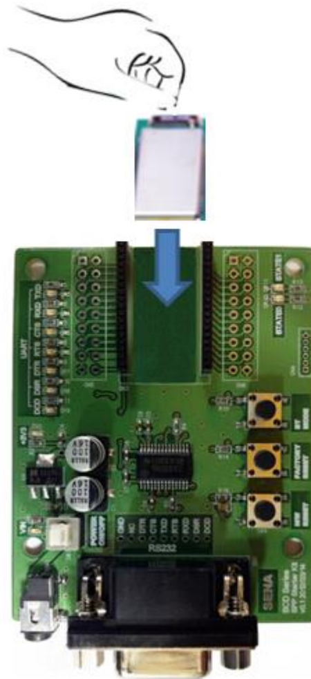
그림 2-2 Parani-BCDx10을 개발 보드에 연결
