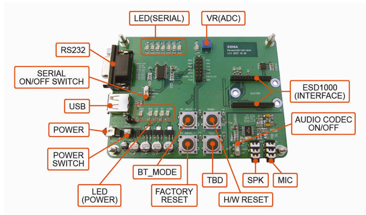
그림 2-1 지그 보드 패널 배치
