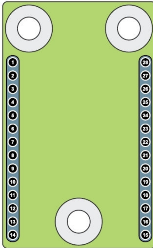
그림 A-1 Parani-ESD의 핀 사양
