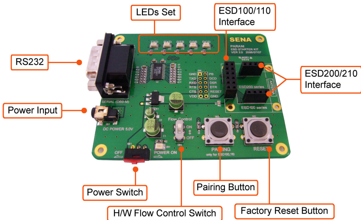
그림 2-1 지그 보드 패널 배치
