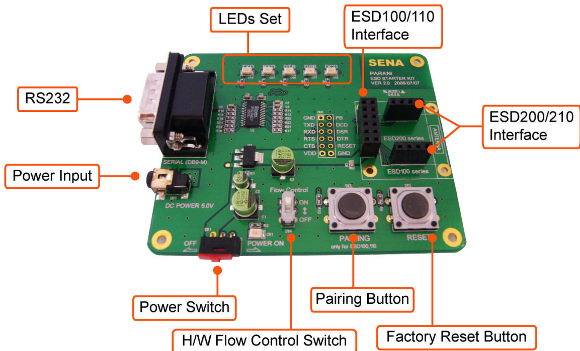
그림 Error! Style not defined.-1 지그 보드 패널 배치
