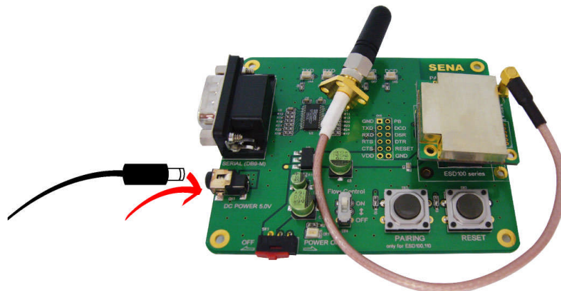
그림 Error! Style not defined. -3 지그 보드에 전원 연결
