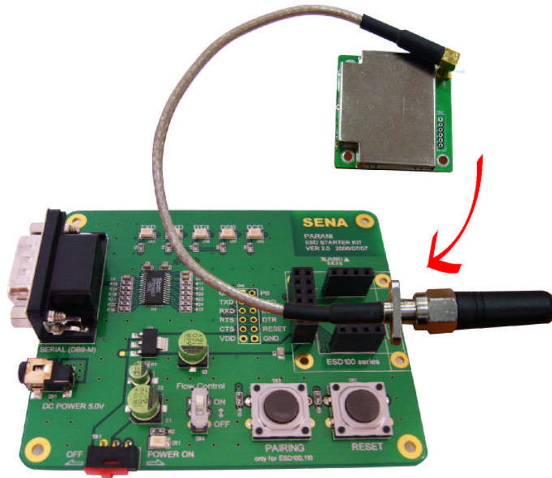
그림 Error! Style not defined. -2 Parani-ESD를 지그 보드에 연결
