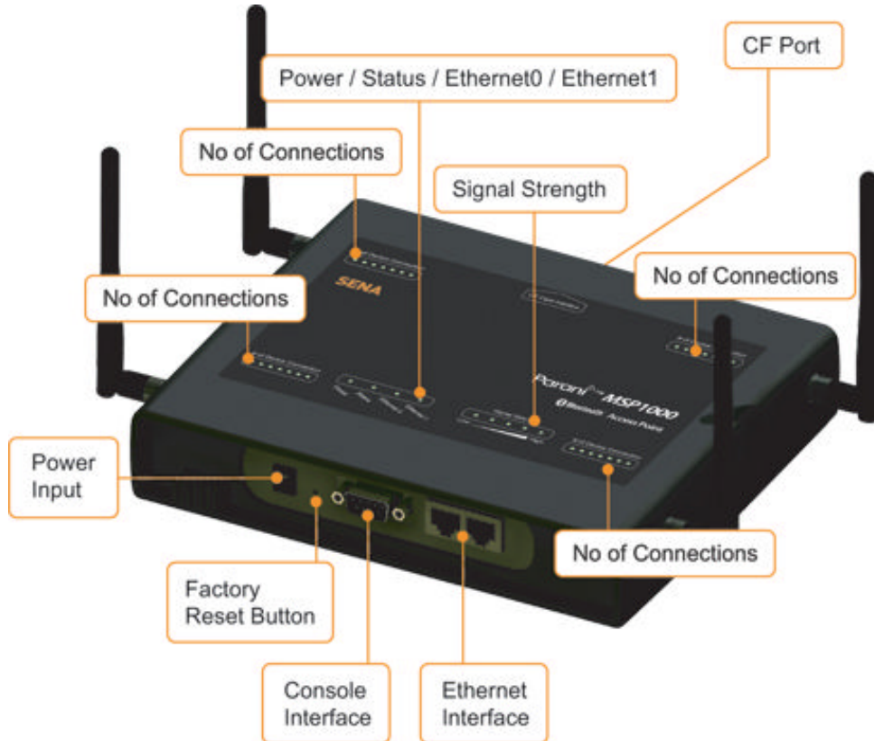
그림 2-1 Parani-MSP1000 외관
