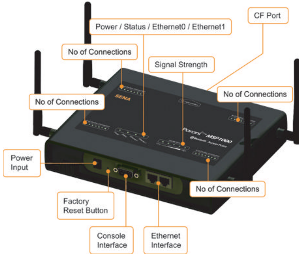
그림 2-1 Parani-MSP1000 외관
