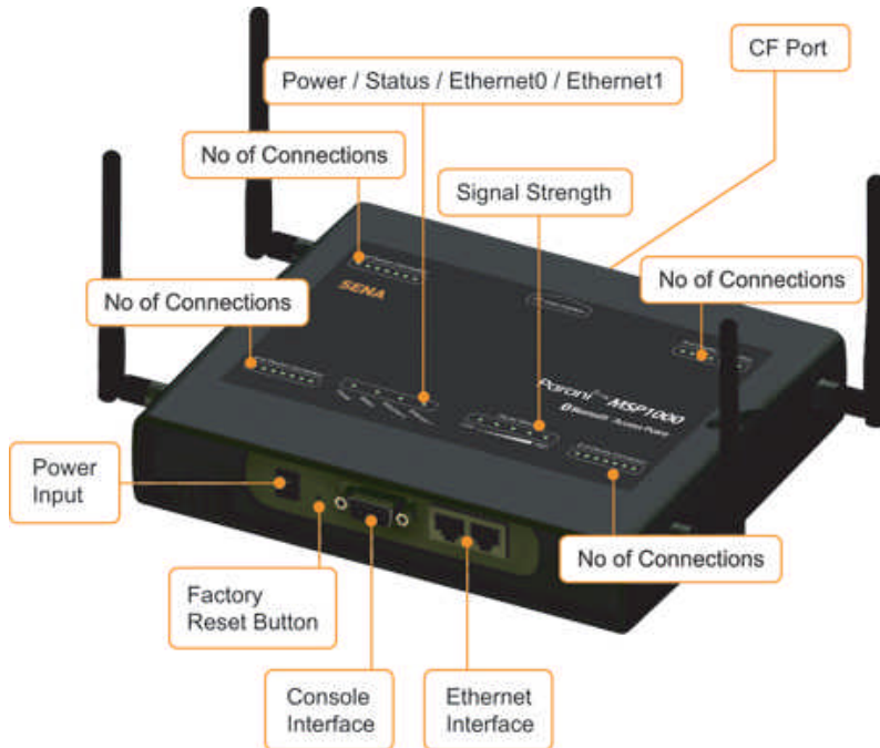
그림 2-1 Parani-MSP1000 외관
