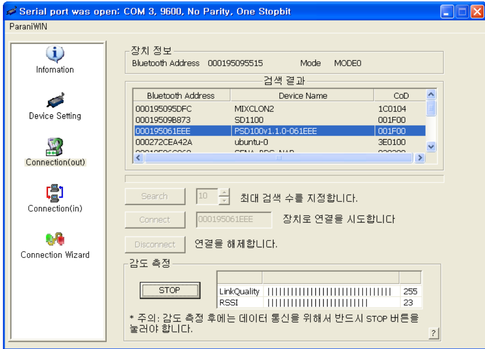
그림 3-8 감도 측정
