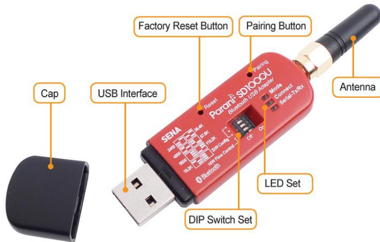
그림 2-1 SD1000U 패널 배치
