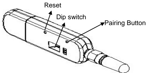
그림 3-1 SD1000U 딥 스위치
