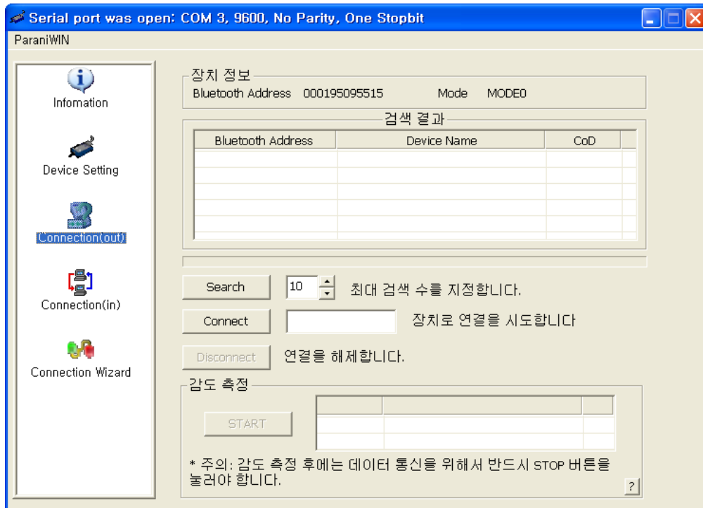
그림 3-7 Connection(out) 화면
