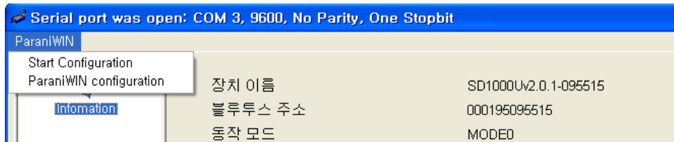
그림 3-5 ParaniWIN 메뉴
