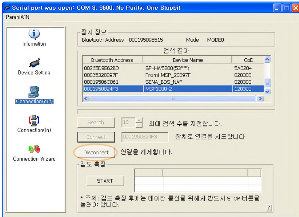
그림 3-3 Disconnect 화면
