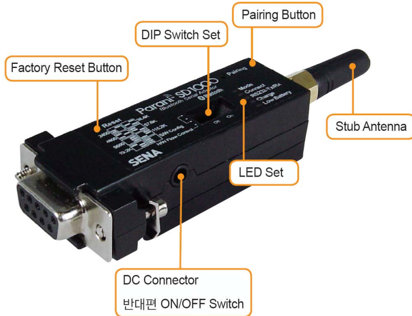
그림 2-1 SD1000 패널 배치
