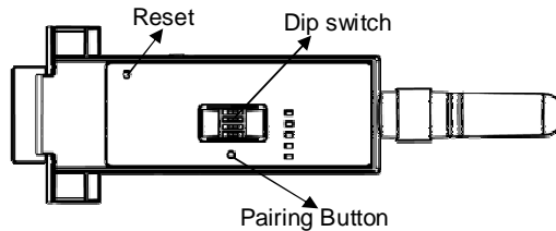
그림 3-1 SD1000 DIP 스위치
