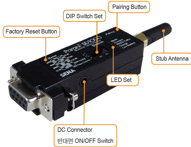
그림 2-1 SD1000 패널 배치
