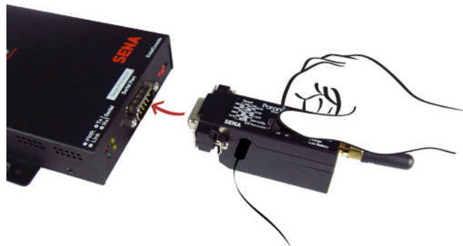
그림 2-3 시리얼 장치에 SD1000 연결
