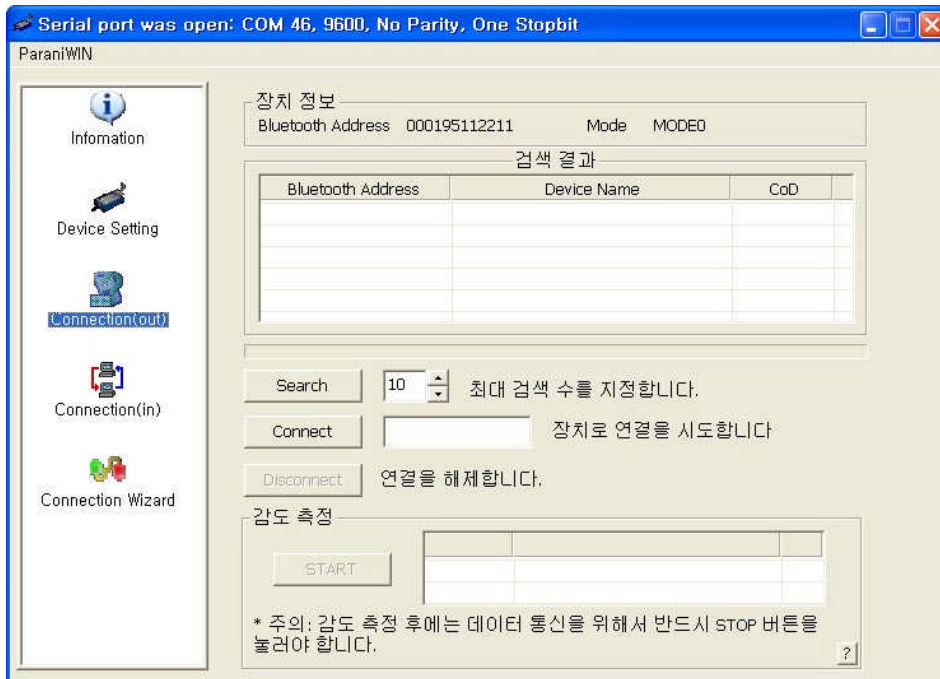
그림 3-7 Connection(out) 화면
