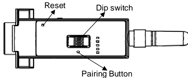
그림 3-1 SD1000 딥 스위치
