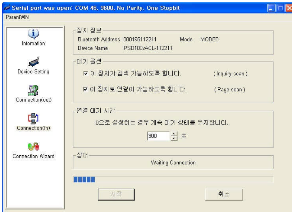
그림 3-9 Connection(in) 화면
