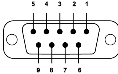
그림 A-1 DB-9 핀 배열
