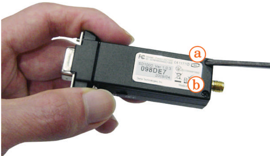
그림 Error! Style not defined.-5 SD1000 후면 덮개 제거
