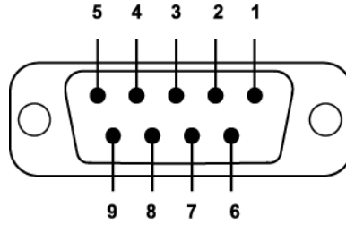
그림 A-1 DB-9 핀 배열
