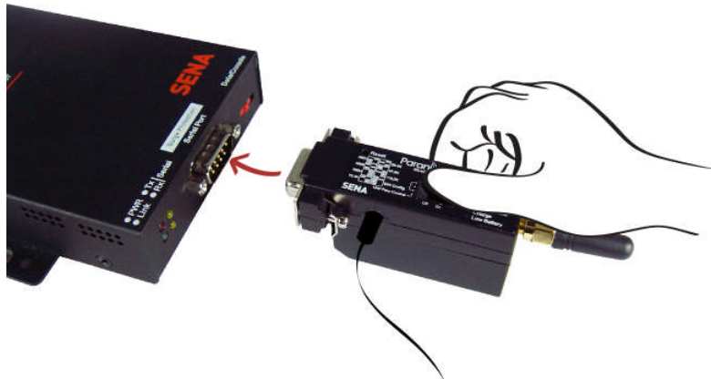
그림 Error! Style not defined.-3 시리얼 장치에 SD1000 연결
