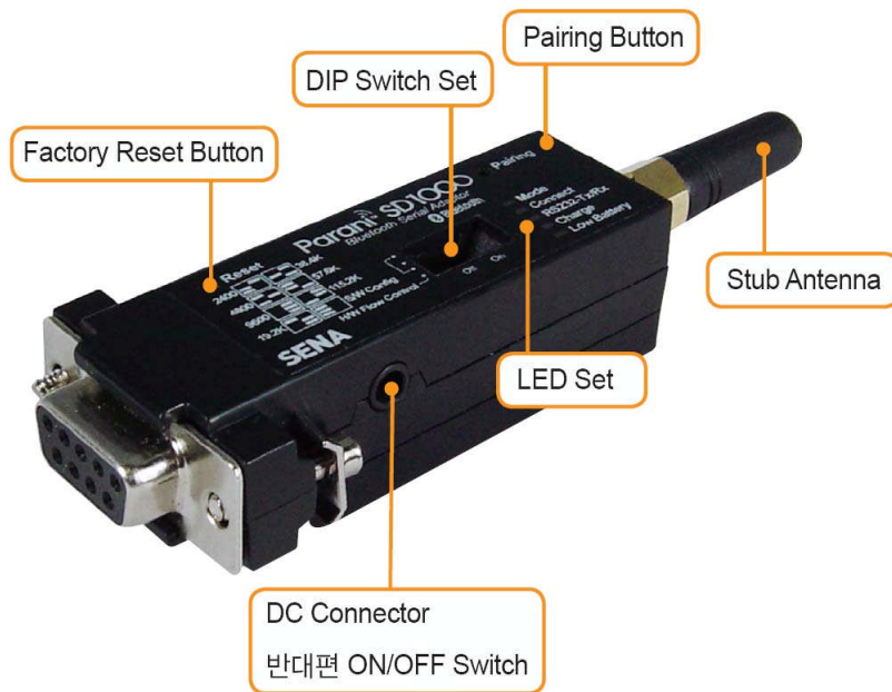
그림 Error! Style not defined. -1 SD1000 패널 배치
