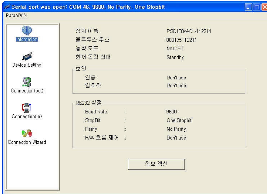
그림 3-4 Information 화면
