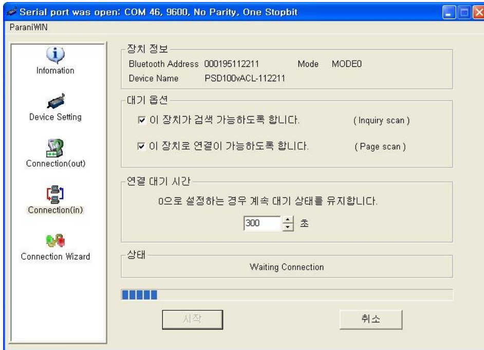
그림 3-9 Connection(in) 화면
