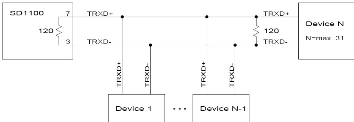
그림 A-3 RS485 시리얼 배선도
