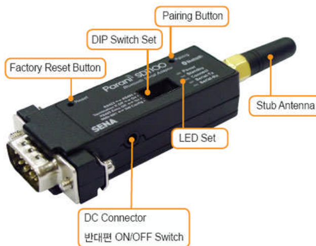
그림 Error! Style not defined.-2 SD1100 패널 배치
