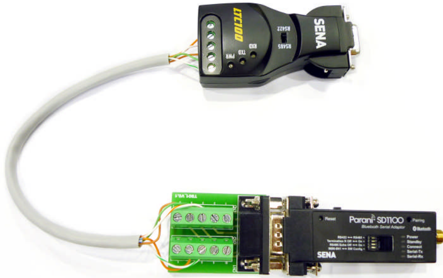
그림 3-15 펌웨어 업데이트 키트
