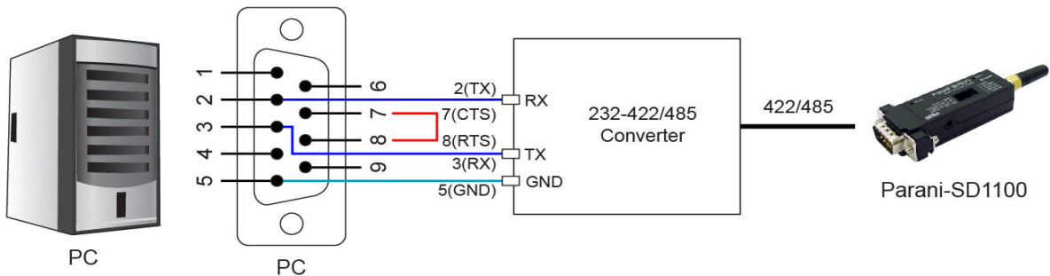
그림 3-14 펌웨어 업데이트를 위한 시리얼 배선
