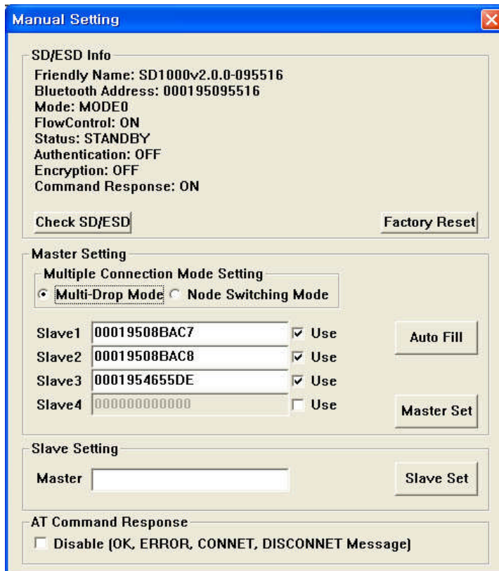
그림 3-12 Manual Setting 화면
