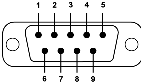
그림 A-1 DB-9 핀 배열
