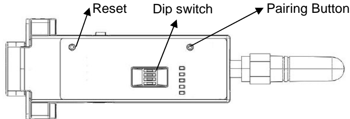
그림 3-1 SD1100 DIP 스위치
