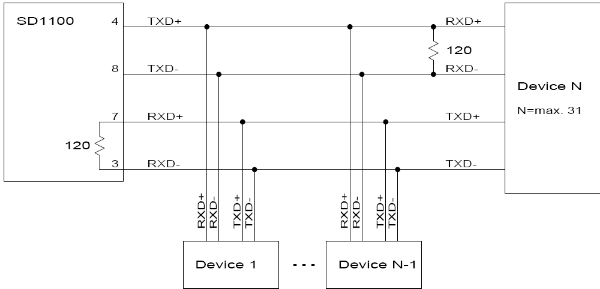
그림 A-2 RS422 시리얼 배선도
