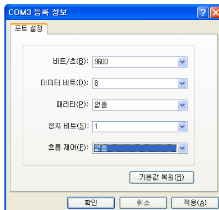
그림 3-16 HyperTerminal
