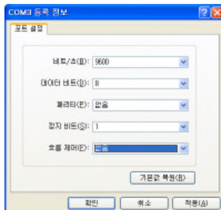
그림 3-16 HyperTerminal
