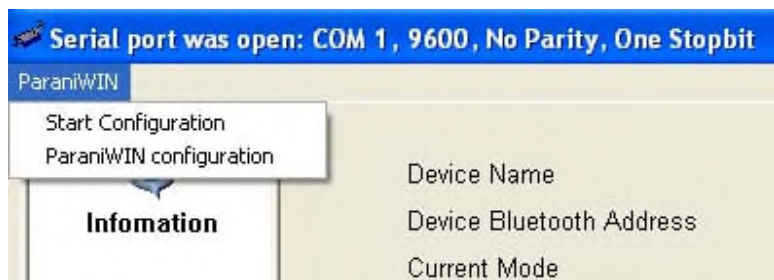
그림 3-5 ParaniWIN 메뉴
