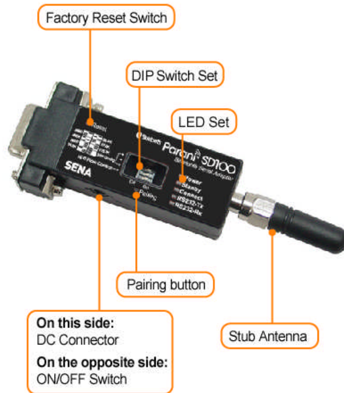
그림 Error! Style not defined. -1 Parani-SD100 패널 배치
