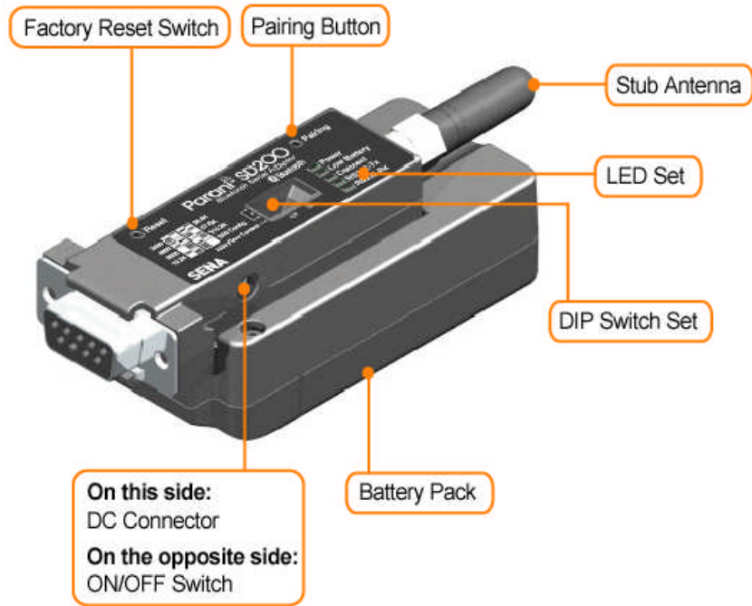
그림 Error! Style not defined. -2 Parani-SD200 패널 배치
