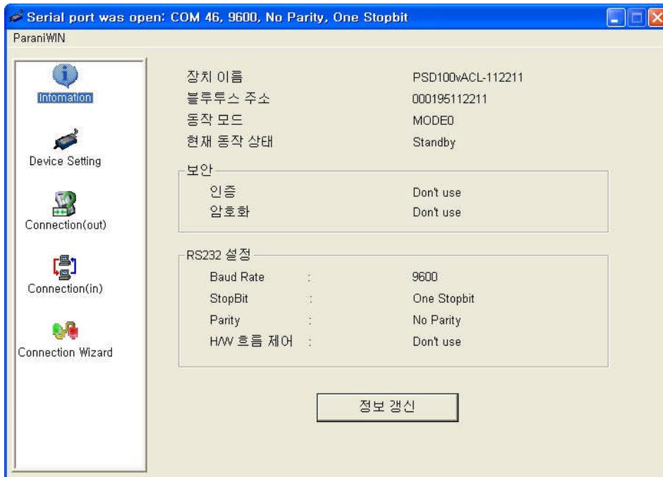
그림 3-4 Information 화면
