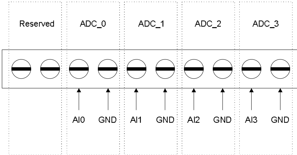
그림 6-2 외부 아날로그 입력용 터미널 블록
