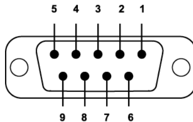
그림 8-1 DB-9 핀 배열
