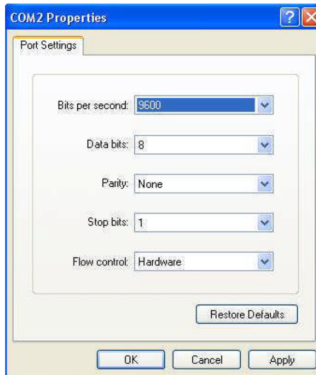
그림 2-8 HyperTerminal 시리얼 포트 설정
