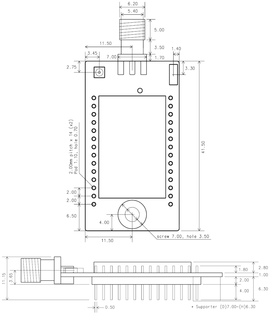
그림 11-1 치수
