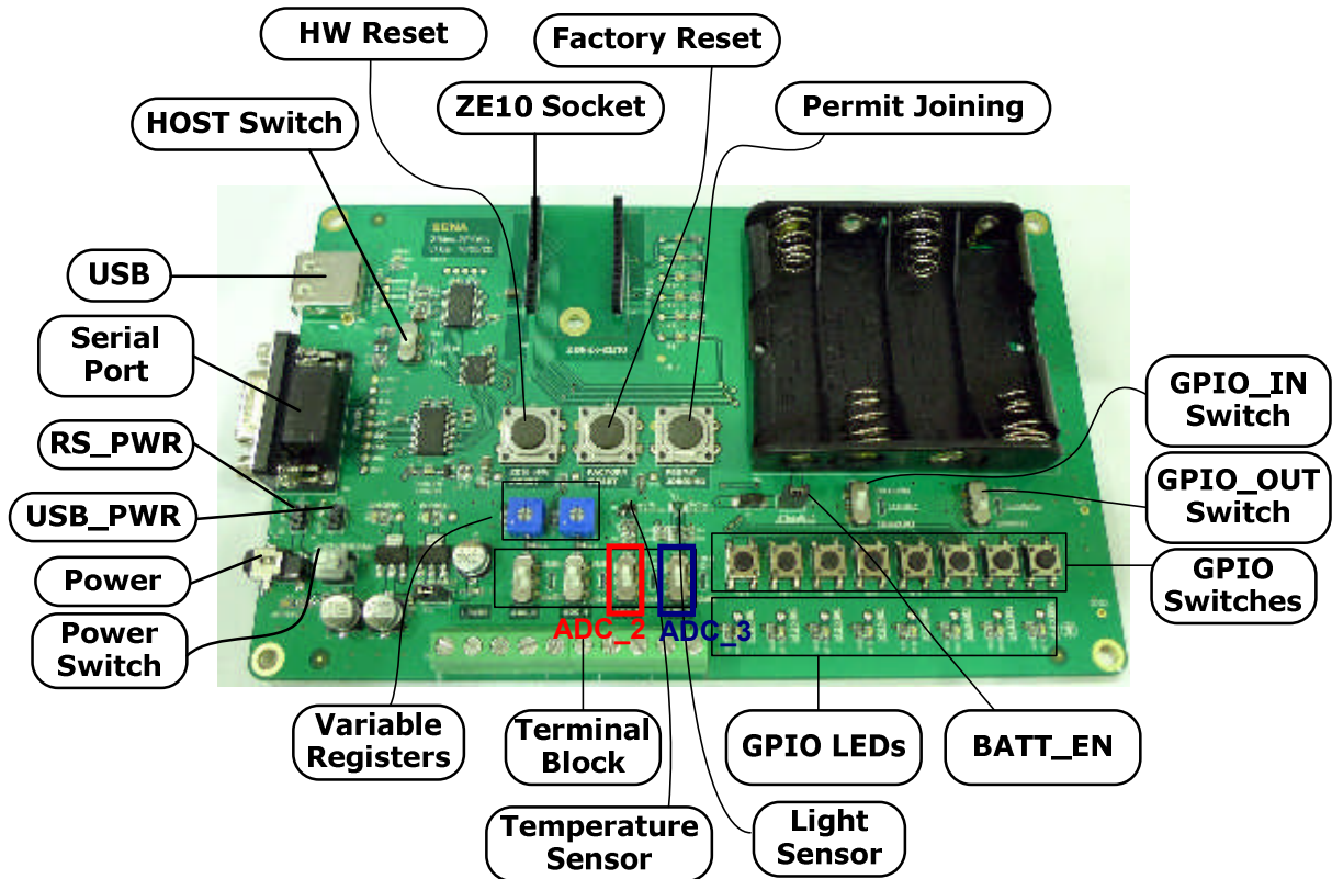
그림 6-6 하드웨어 설정
