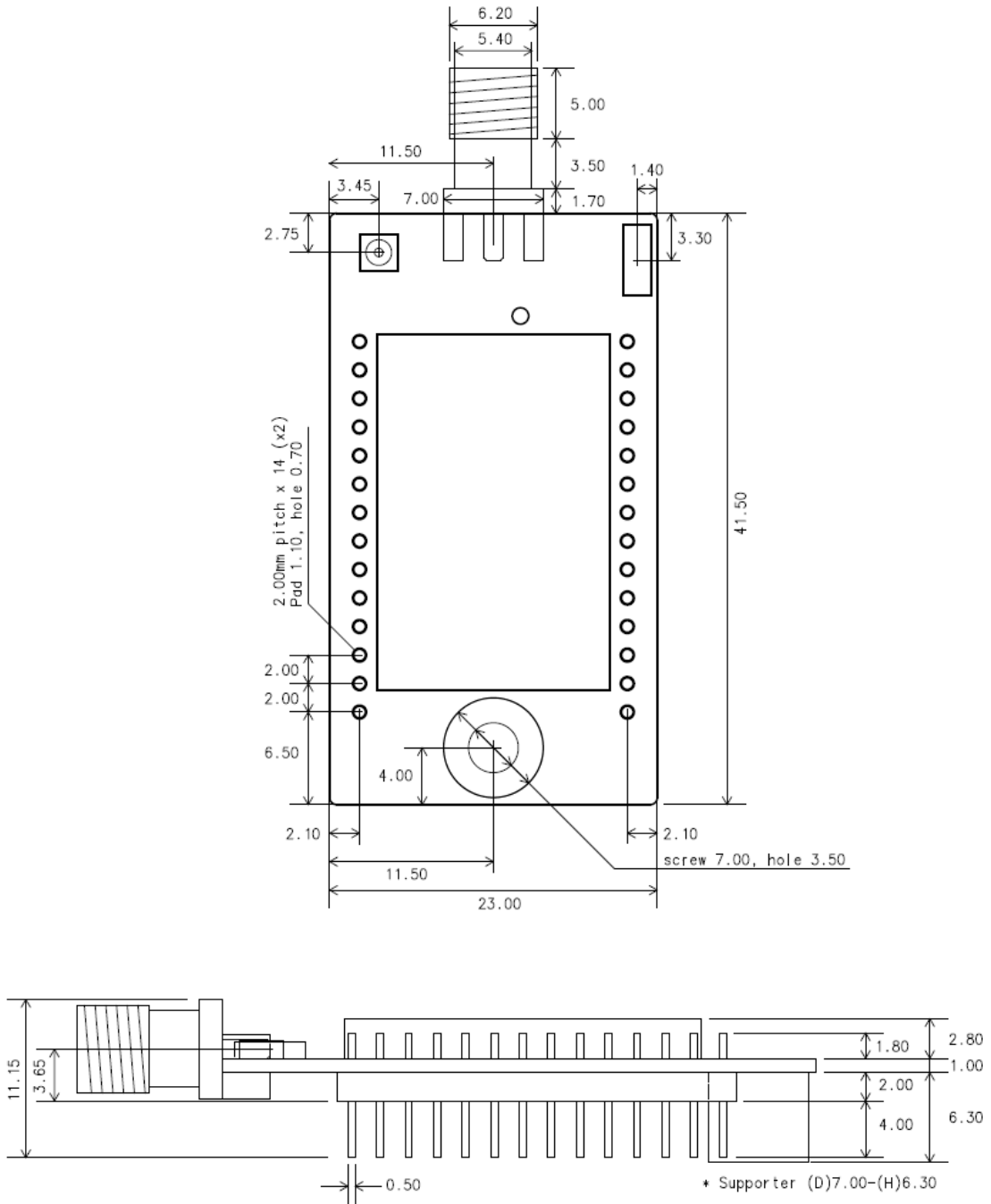
그림 12-1 치수
