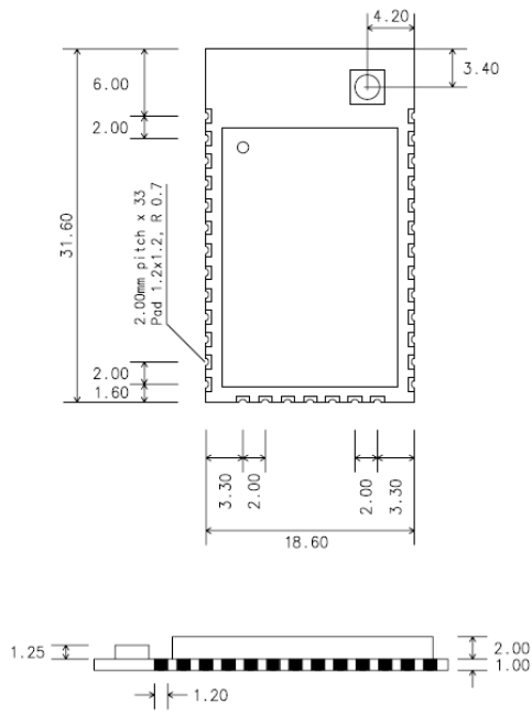
그림 11-4 ProBee-ZE20SSU 치수
