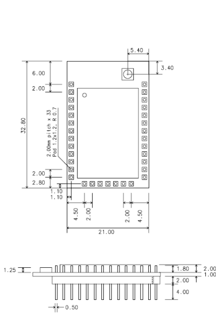
그림 11-1 ProBee-ZE20SDU 치수
