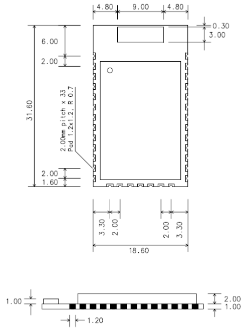
그림 11-5 ProBee-ZE20SSC 치수
