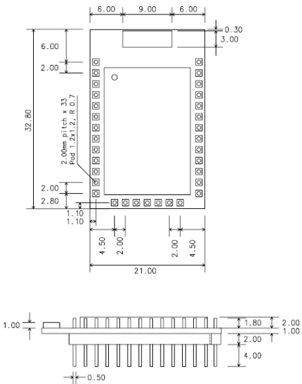
그림 11-3 ProBee-ZE20SDC 치수
