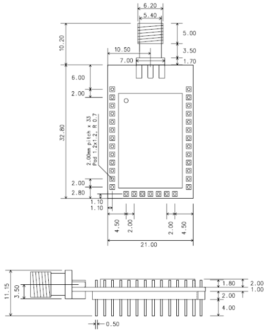
그림 11-2 ProBee-ZE20SDS 치수
