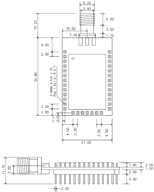
그림 11-2 ProBee-ZE20SDS 치수
