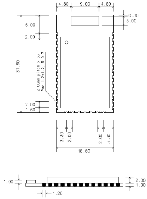
그림 11-5 ProBee-ZE20SSC 치수
