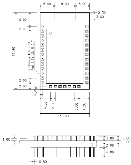
그림 11-3 ProBee-ZE20SDC 치수
