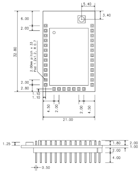
그림 11-1 ProBee-ZE20SDU 치수
