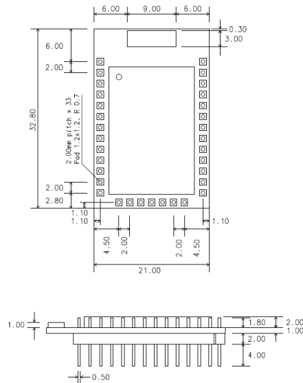
그림 12-3 ProBee-ZE20SDC 치수
