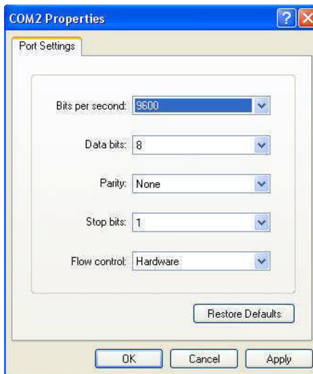
그림 2-3 HyperTerminal 시리얼 포트 설정
