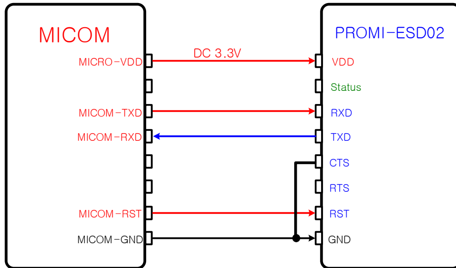
그림 3-8 TTL Level 3.3V FW OFF ESD02 결선도
