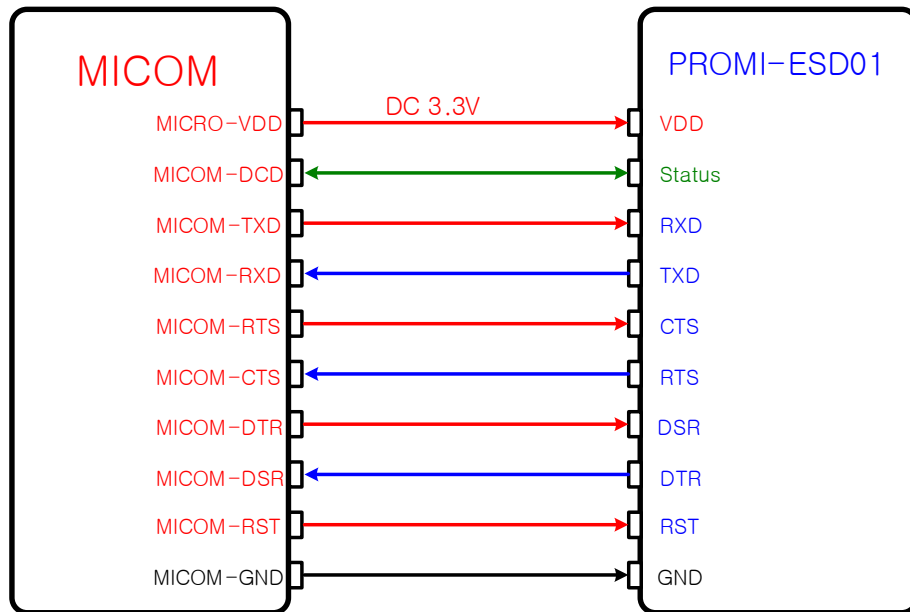
그림 3-3 TTL Level 3.3V ESD01 결선도
