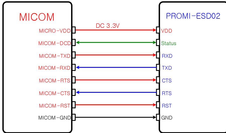
그림 3-7 TTL Level 3.3V ESD02 결선도
