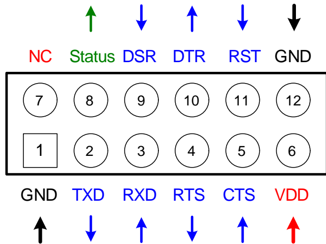
그림 3-1 ESD01 핀 사양
