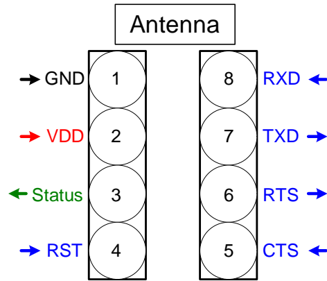
그림 3-2 ESD02 핀 사양
