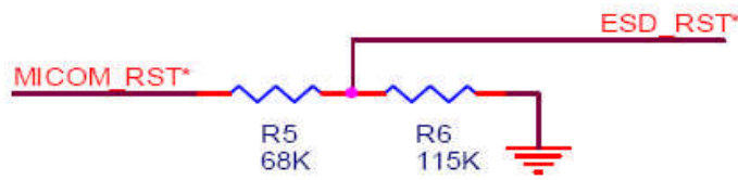
그림 3-6 Reset 사용시 ESD 결선도
