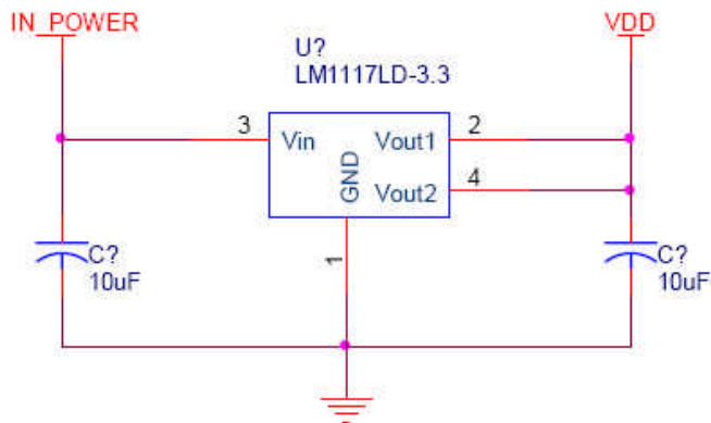
그림 5-1 1117 시리즈를 이용한 일반적인 3.3V 출력 회로
