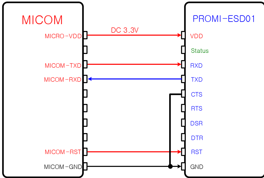
그림 3-4 TTL Level 3.3V FW OFF ESD01 결선도
