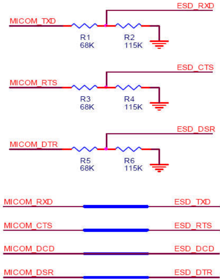
그림 3-5 TTL Level 5V ESD01 결선도
