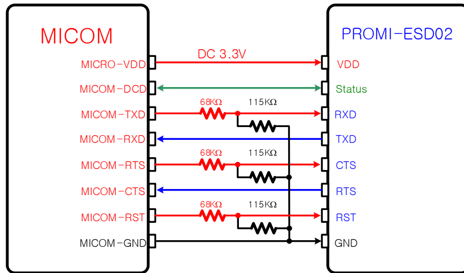
그림 3-9 TTL Level 5V ESD02 결선도
