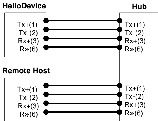
그림 A-5 스트레이트 이더넷 케이블을 사용한 이더넷 연결
