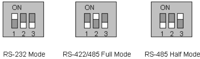
그림 4-14 시리얼 통신 형식과 DIP 스위치 설정(PS110/410)
