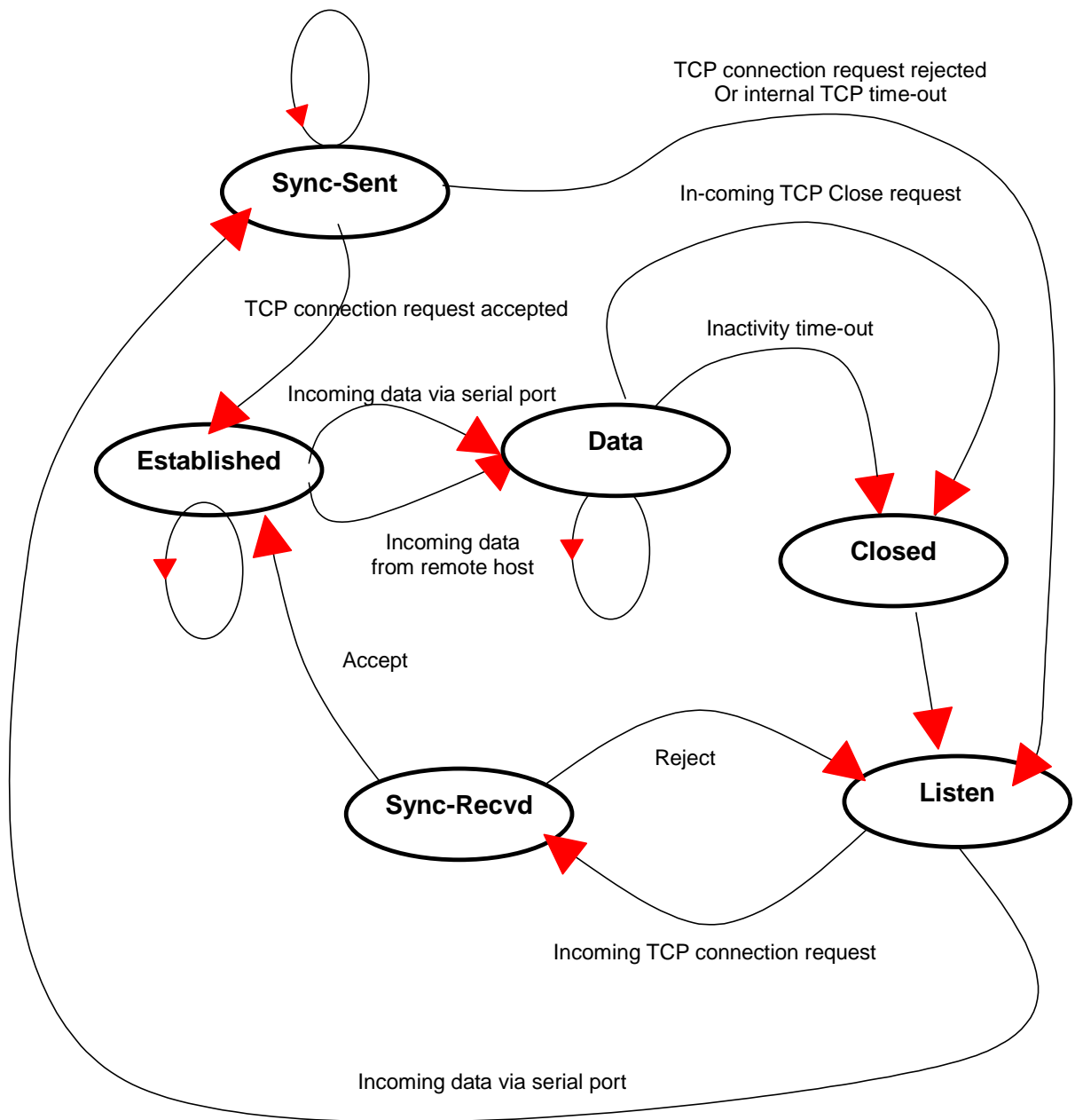
그림 4-5 TCP모드의 상태전이도
