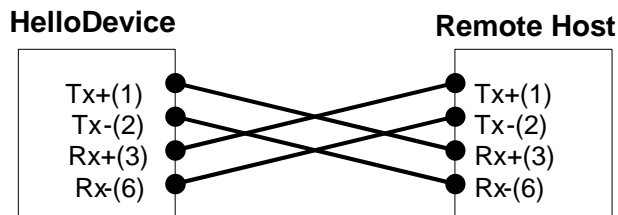
그림 A-4 크로스오버 이더넷 케이블을 사용한 이더넷 직접 연결
