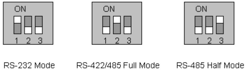
그림 A-3 Serial communication type and DIP switch configuration
