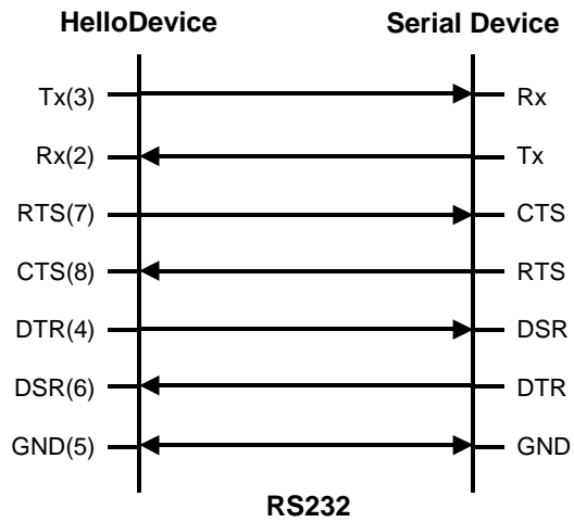
그림 A-6 RS232 시리얼 배선도
