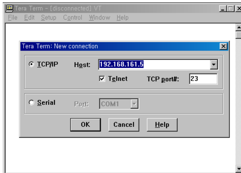
그림 2-17 Telnet 프로그램 설정 예제 (TeraTerm Pro)
