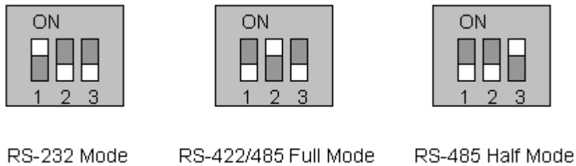
그림 A-1 Serial communication type and DIP switch configuration
