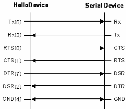
그림 A-5 RS232 시리얼 배선도
