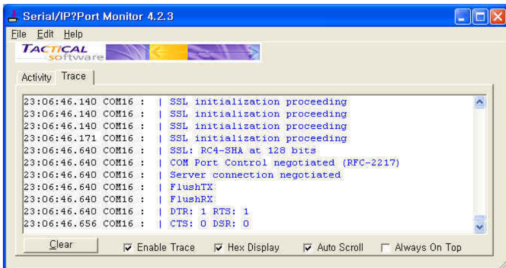
그림 A-18 Serial/IP Trace Window
