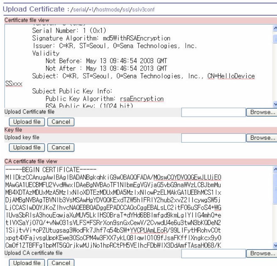
그림 4-12 인증서 업로드
