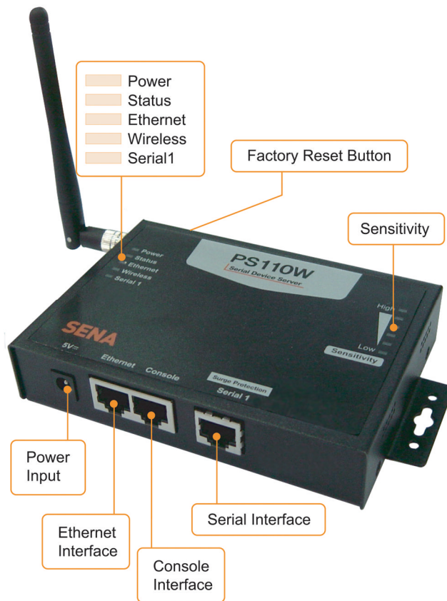
그림 2-1 PS110W의 패널 레이아웃
