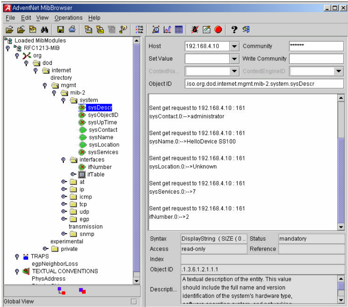
그림 3-8 SNMP 브라우저를 사용한 Pro Series SNMP 에이전트의 MIB-II OID 표시 (AdventNet MIB브라우저)
