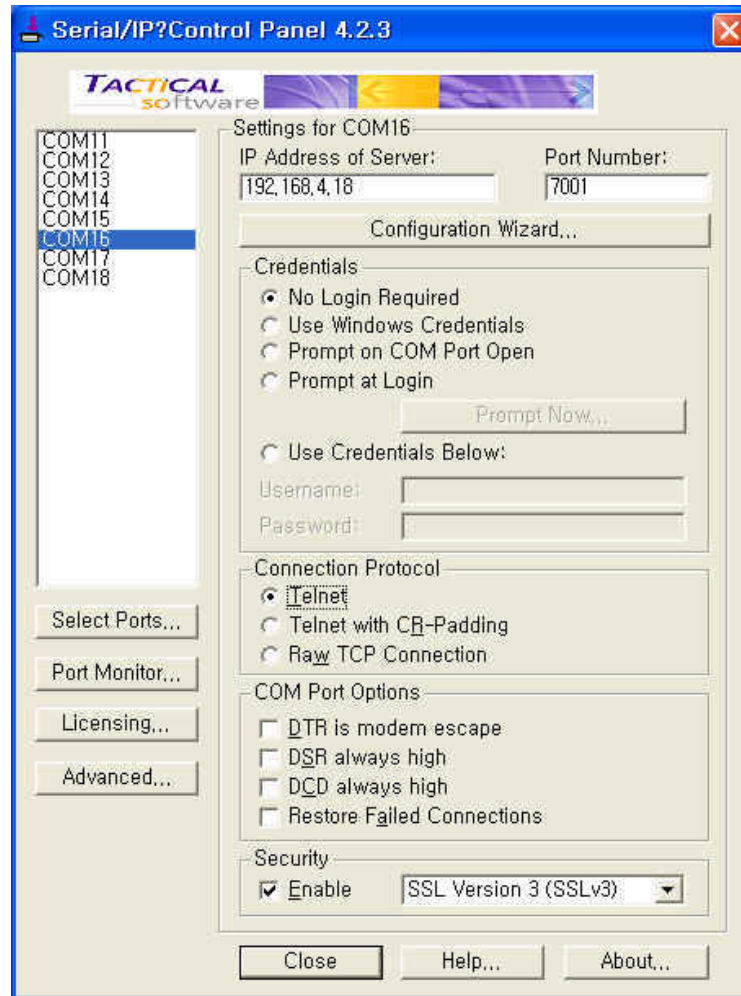
그림 A-16 Serial/IP Control Panel에서 파라미터 설정
