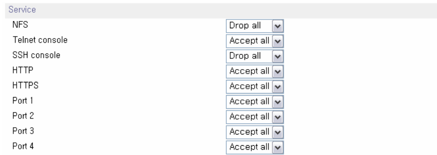
그림 3-14 각 service 및 시리얼 port 에 대한 IP 필터링 설정
