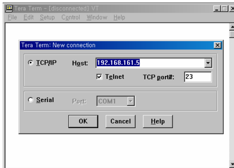
그림 2-8 Telnet 프로그램 설정 예제 (TeraTerm Pro)
