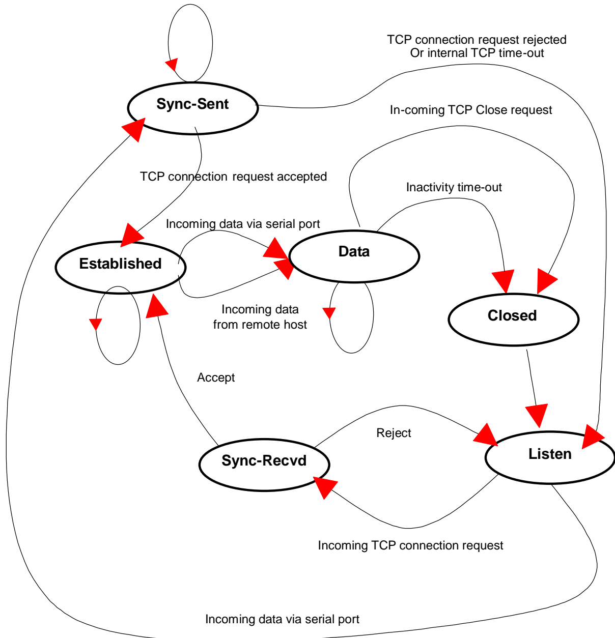
그림 4-5 TCP모드의 상태전이도
