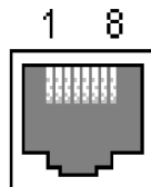
그림 A-2 RJ-45 커넥터의 핀 배치
