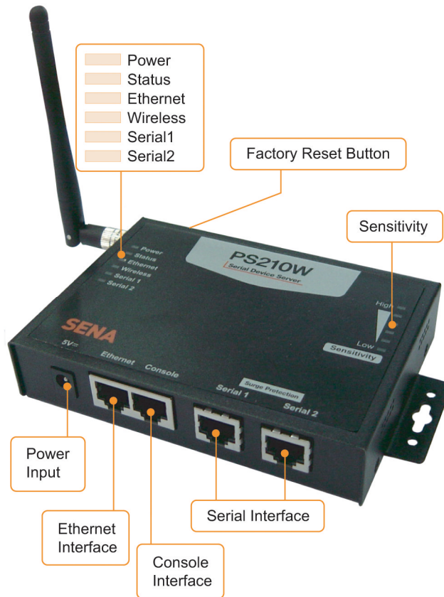
그림 2-2 PS210W의 패널 레이아웃
