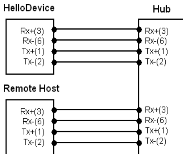
그림 A-4 스트레이트 이더넷 케이블을 사용한 이더넷 연결
