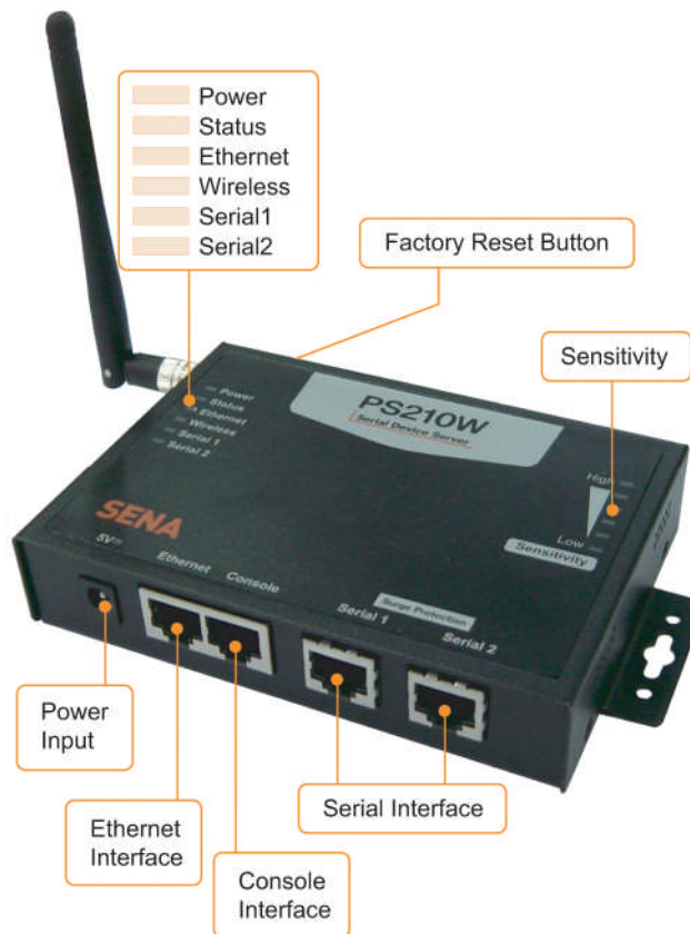
그림 2-2 PS210W의 패널 레이아웃
