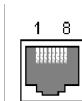
그림 A-2 RJ-45 커넥터의 핀 배치
