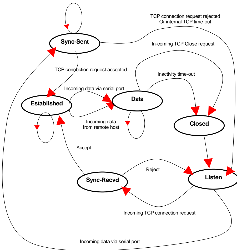
그림 4-5 TCP모드의 상태전이도
