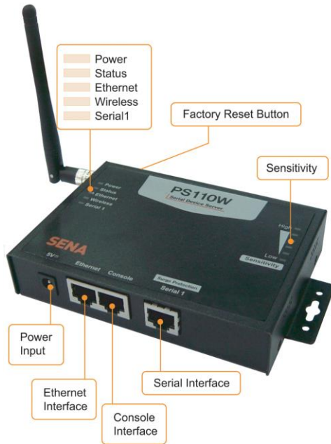
그림 2-1 PS110W의 패널 레이아웃
