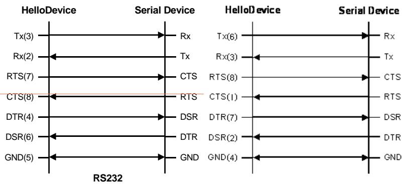
그림 A-5 RS232 시리얼 배선도
