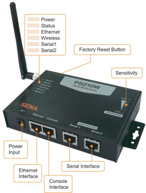
그림 2-22. PS210W의 패널 레이아웃
