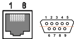
그림 A-2 DB9-RJ45 커넥터의 핀 배치
