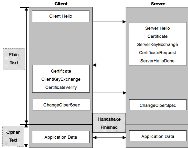
그림 4-11 일반적인 SSL 핸드셰이크 프로세스
