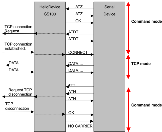
그림 4-7 모뎀 에뮬레이션 모드의 명령/데이터 흐름의 전형적인 예
