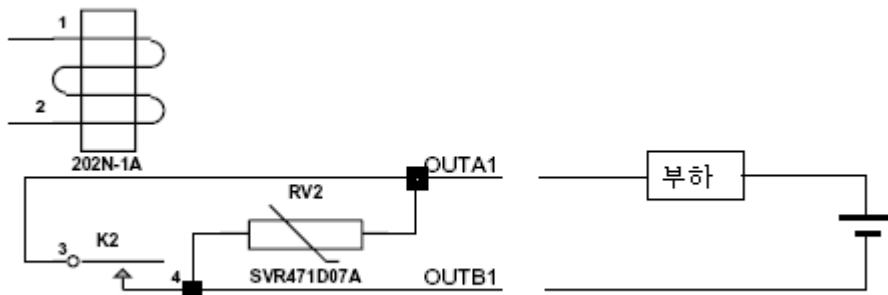
그림 4-6 Digital Output Port 연결
