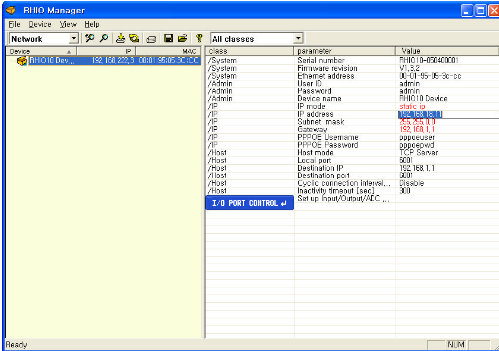
그림 3-3 네트워크 설정 예
