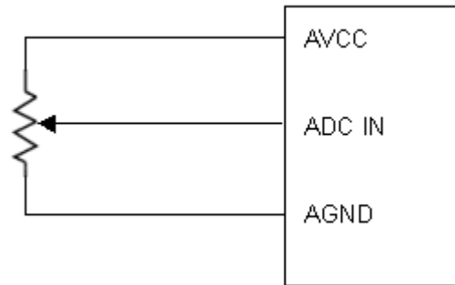
그림 4-9 Potentionmeter 사용시의 연결
