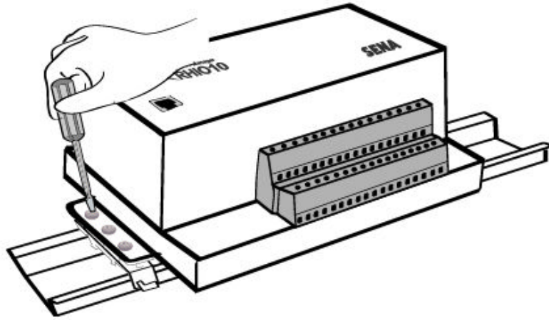
그림 2-4. DIN 레일에 Rhio10 설치 및 부착
