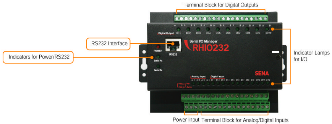
그림 2-1. Rho232의 패널 배치
