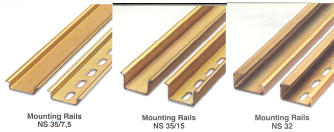
그림 2-2. DIN 레일 거취형 키트 치수 및 적용되는 DIN 레일
