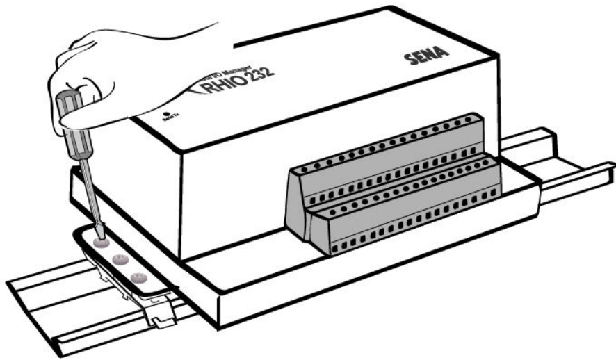
그림 2-4. DIN 레일에 Rhio232 설치 및 부착
