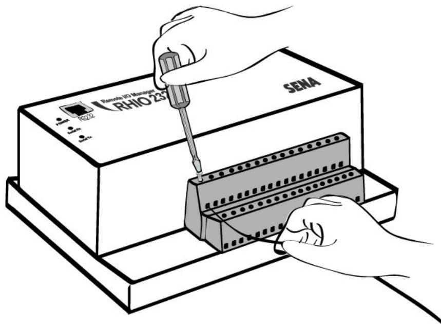
그림 2-5. Rhio232 에 전원 연결
