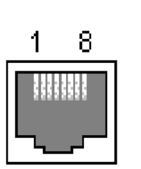
그림 A-1 RJ45 커넥터의 핀 배치
