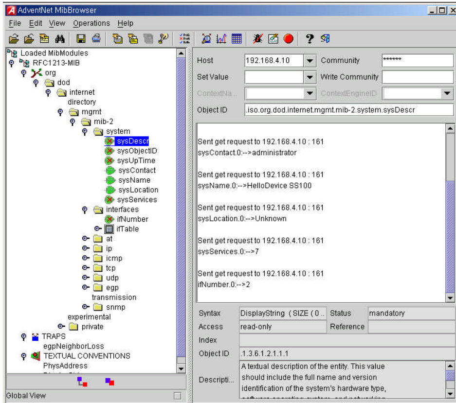
그림 3-3 SNMP 브라우저를 사용한 STS 시리즈 SNMP 에이전트의 MIB-II OID 브라우저 (AdventNet MIB 브라우저)
