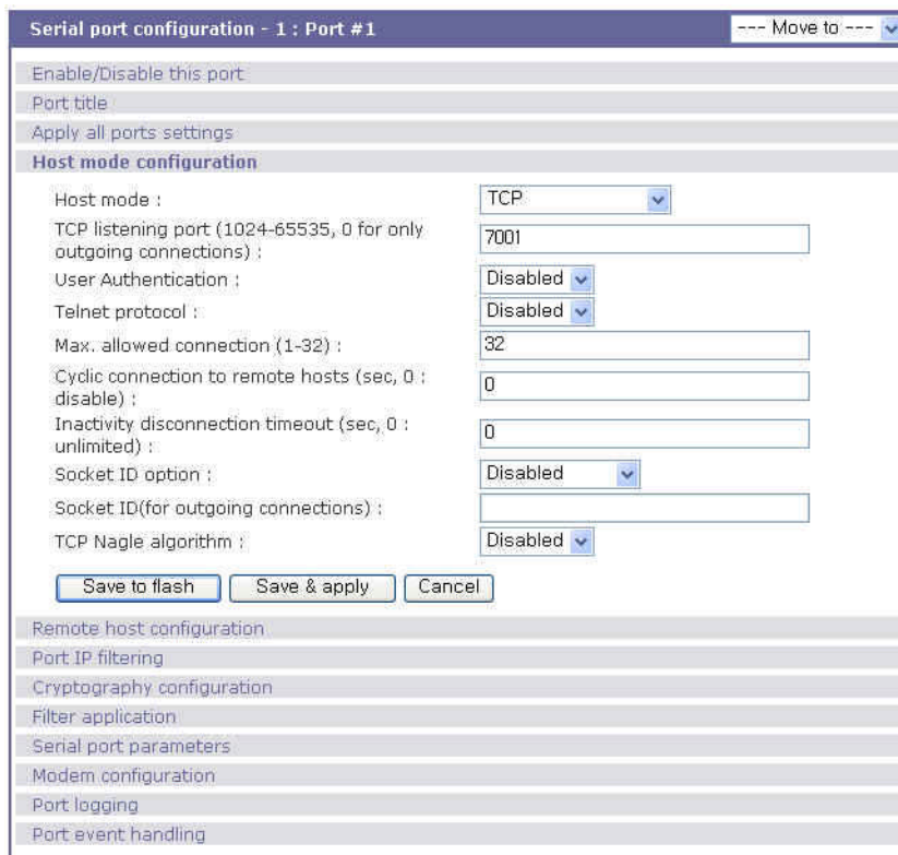
그림 4-5 호스트 모드 환경설정
