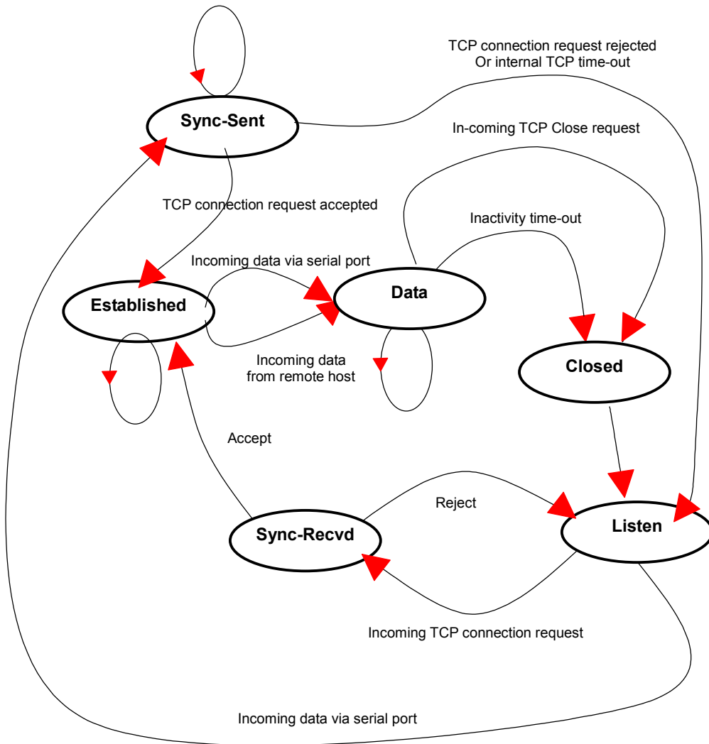
그림 4-6 TCP모드의 상태전이도
