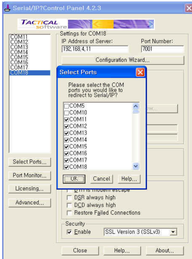
그림 A-13 Serial/IP Control Panel에서 포트들을 선택
