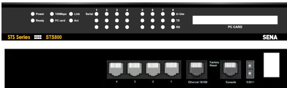
그림 2-1 STS800의 패널 레이아웃
