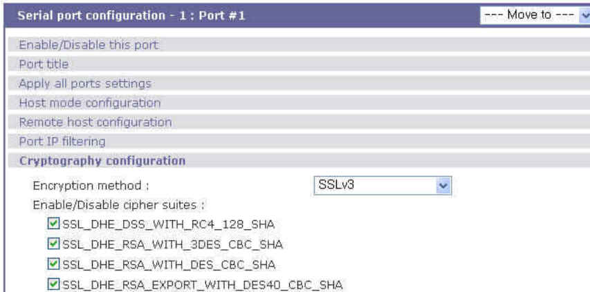
그림 A-12 암호기법 설정( Cryptography configuration)
