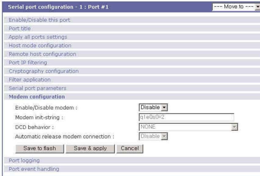
그림 4-16 모뎀 구성
