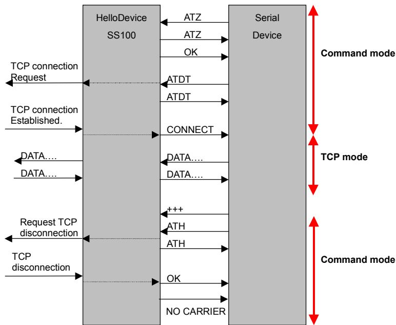
그림 4-7 모뎀 에뮬레이션 모드의 명령/데이터 흐름의 전형적인 예
