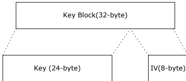
그림 4-13 키 유도
