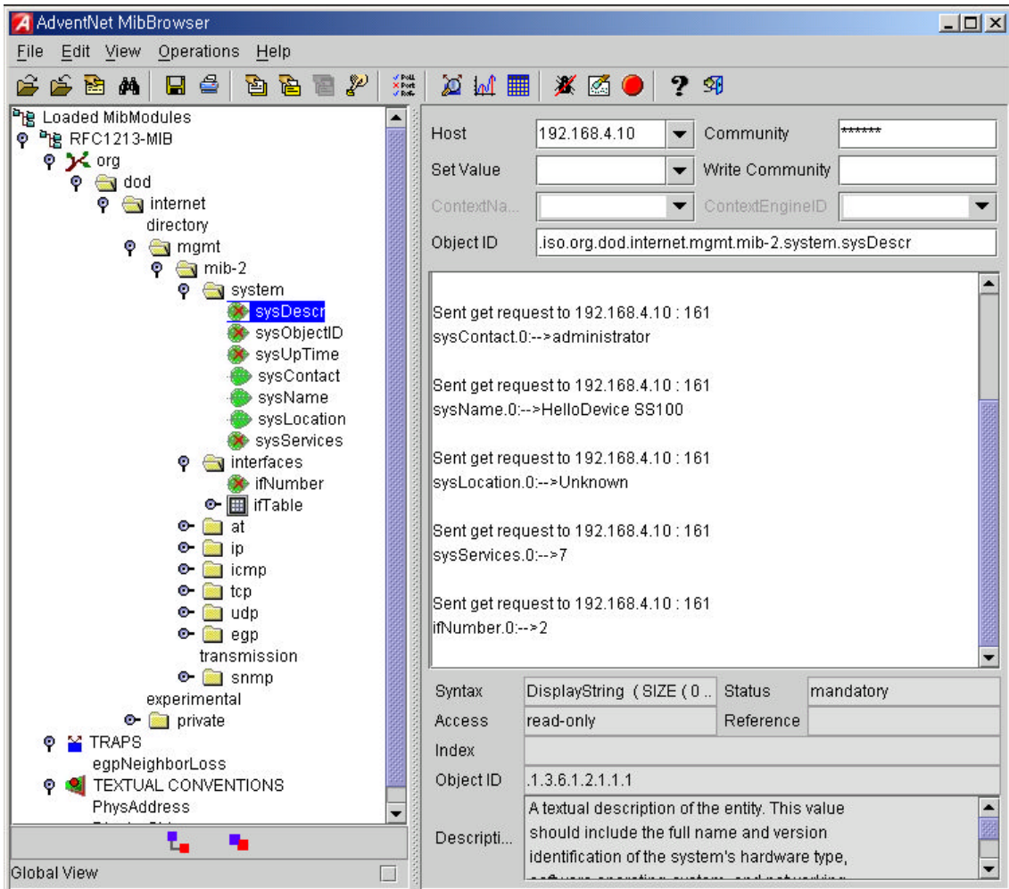
그림 3-3 SNMP 브라우저를 사용한 STS 시리즈 SNMP 에이전트의 MIB-II OID 브라우저 (AdventNet MIB브라우저)
