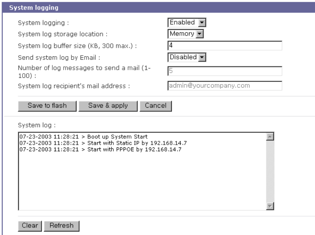
그림 6-2 시스템 로그 설정 및 보기
